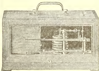
Richard-féle barográf.
