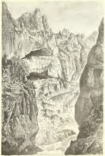
Részletek a St-Kanzian melletti Reka folyó földalatti barlangjaiból.
