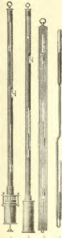
1. Fortin-féle barométer. — 2. Kappeller-féle barométer. — 3. és 4. Gay-Lussac-féle barométer.
