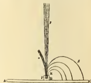
Becquerel-sugarak mágneses térben. A sugarak a P ólomcsészében levő R rádiumbromidból indulnak ki, a mágnes északi sarkát a rajz síkja elzárja, a déltől mögötte kell gondolnunk, AO fényérzékeny lemez.
