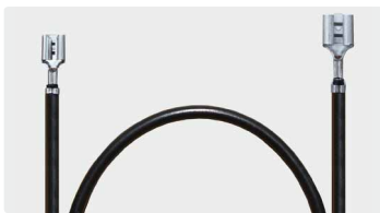
Cable lug 6.3 : cable lug 4.8. Cable 500 mm. Cable type 1
