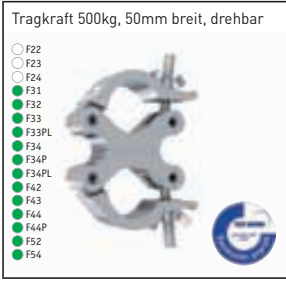
Trussaufnehmer (für 50mm Truss) 8231 43,00 €
