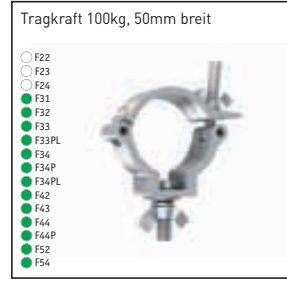
Trussaufnehmer 812 10,50 €
