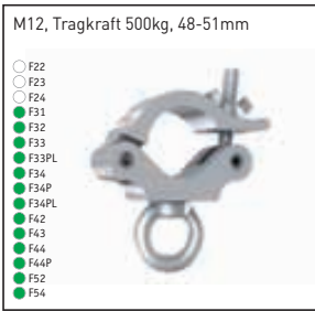
Trussaufnehmer mit Öse 5033 27,00 €
