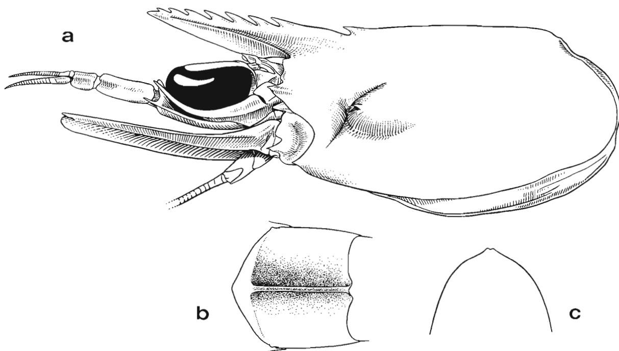
FIG. 20. — Metapenaeopsis distincta (de Man, 1907), ♀ 13,7 mm, Nouvelle-Calédonie, LAGON, st. 995 (MNH-Na 12678) : a, partie antérieure du corps; b-c, troisième segment abdominal, vue dorsale et coupe transversale.
