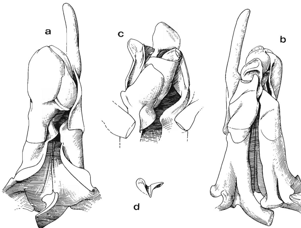
FIG. 22. — Metapenaeopsis distincta (de Man, 1907), ♂ 7,3 mm, Nouvelle-Calédonie, LAGON, st. 590 (MNHN-Na 12677). Pétaσμα : a, vue ventrale; b, vue dorsale; c, vue ventrale de la partie distale, valves écartées; d, vue antérieure de l'extrémité de l'élément distoventral.
