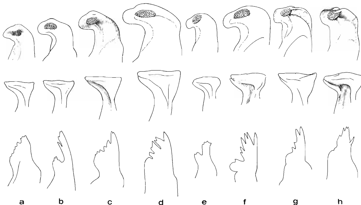
FIG. 46. — Metapenaeopsis hilarula (de Man, 1911). Pétaσμα : de haut en bas, élément distodorsal gauche, vue dorsale; élément distoventral, vue ventrale; extrémité de la valve gauche. a, ♂ 9,6 mm, Philippines, MUSORSTOM 3, st. CP 142 (MNHN-Na 12697); b, ♂ 9,7 mm, îles Seychelles, REVES 2, st. 48 (MNHN-Na 12696); c, Nouvelle-Calédonie, LAGON, st. 468 (MNHN-Na 12700); d, ♂ 13,8 mm, îles Seychelles, REVES 2, st. 23 (MNHN-Na 12692); e, ♂ 8,0 mm, golfe d'Aden, "Meteor", Cruise 5, st. 236 (SMF); f, ♂ 12,1 mm, îles Seychelles, REVES 2, st. 4 (MNHN-Na 12694); g, ♂ 9,4 mm, La Réunion, MD 32, st. CP 43 (MNHN-Na 12690); h, ♂ 10,4 mm, La Réunion, MD 32, st. CP 43 (MNHN-Na 12691).
