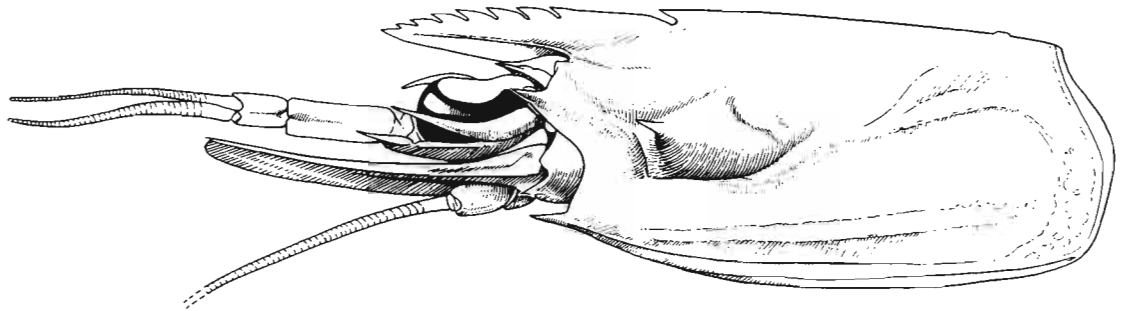
FIG. 79. — Metapenaeopsis wellsi Racek, 1967, ♀ 29,7 mm, Australie, Shark Bay (WAM-358-87) : partie antérieure du corps.
