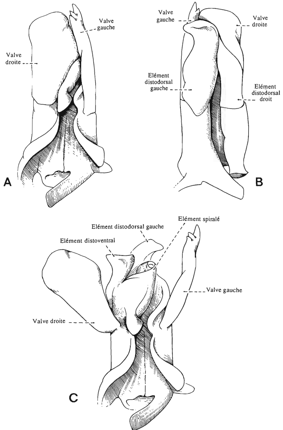
FIG. 2. — Termes utilisés pour la description du pétasma. A, vue ventrale. B, vue dorsale. C, vue ventrale, valves écartées.
