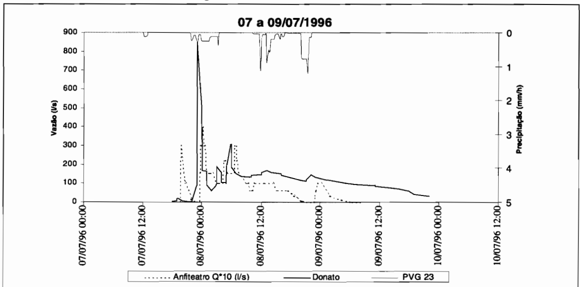
Figura 6.17 - Eventos de 07 a 09 /07/96
