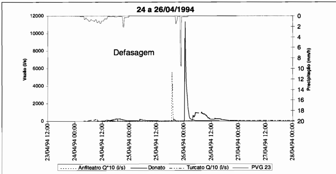
Figura 6.11 - Evento de 24 a26/04/94
