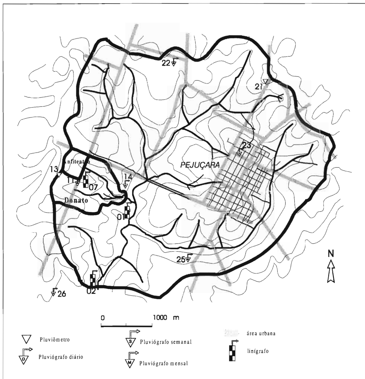
Figura 4.14 - Bacia do Arroio Turcato incluindo bacias do Anfitheatro e Donato
