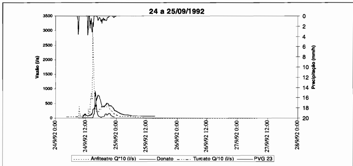
Figura 6.5 - Evento de 24 a 25/09/92
