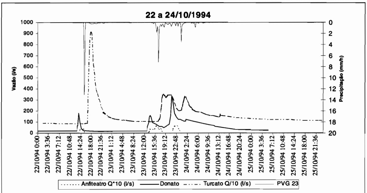
Figura 6.15 - Evento de 22 a 24/10/94
