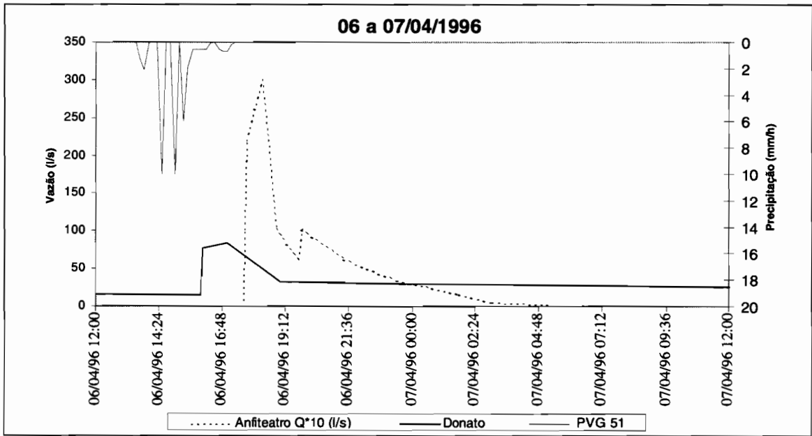
Figura 6.16 - Evento de 06 a 07 /04/96
