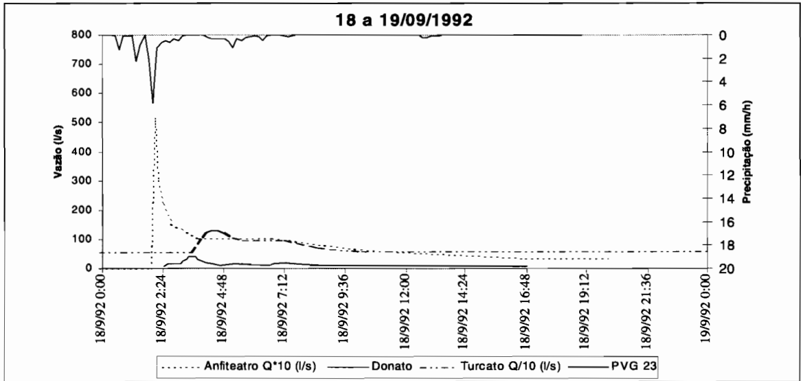
Figura 6.4 - Evento de 18 a 19/09/92
