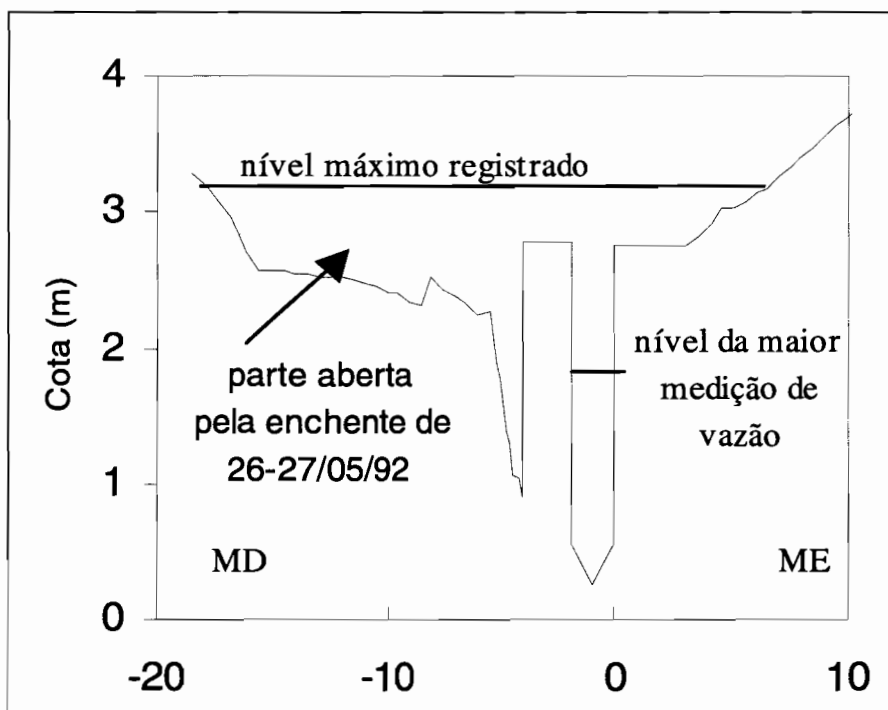
Figura 4.12 - Perfil transversal da estação do Donato após a cheia do dia 27/05/1992
