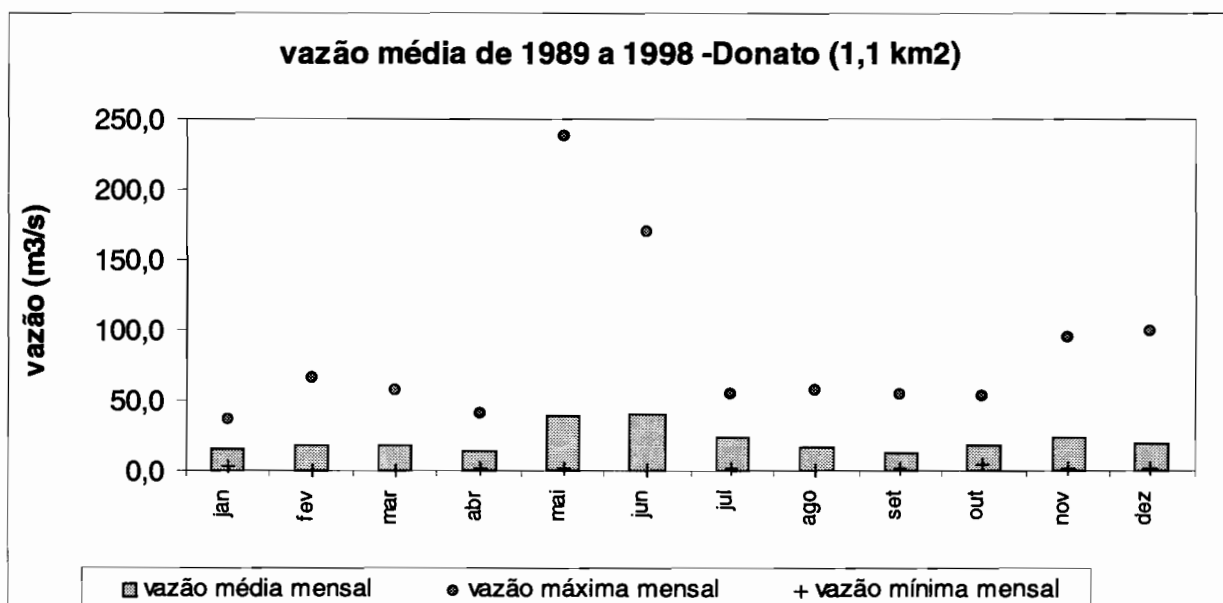
Figura 6.20 - Vazões médias mensais, mín. e máx. mensais das bacias Anfiteatro, Donato e Turcato
