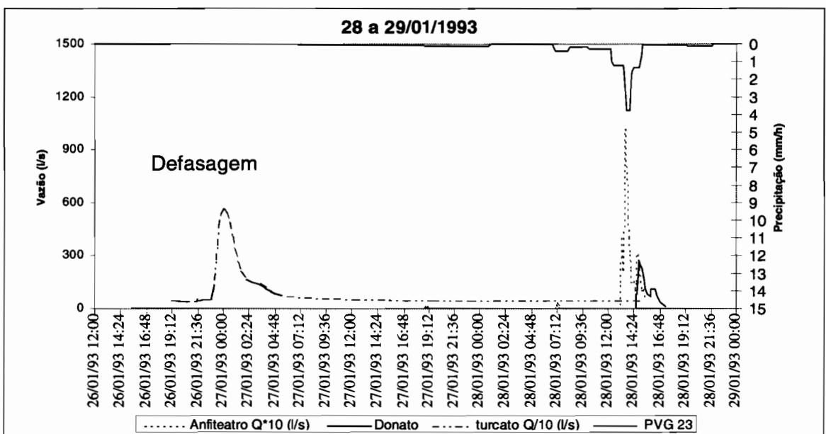
Figura 6.6 - Evento de 28 a 29/01/93
