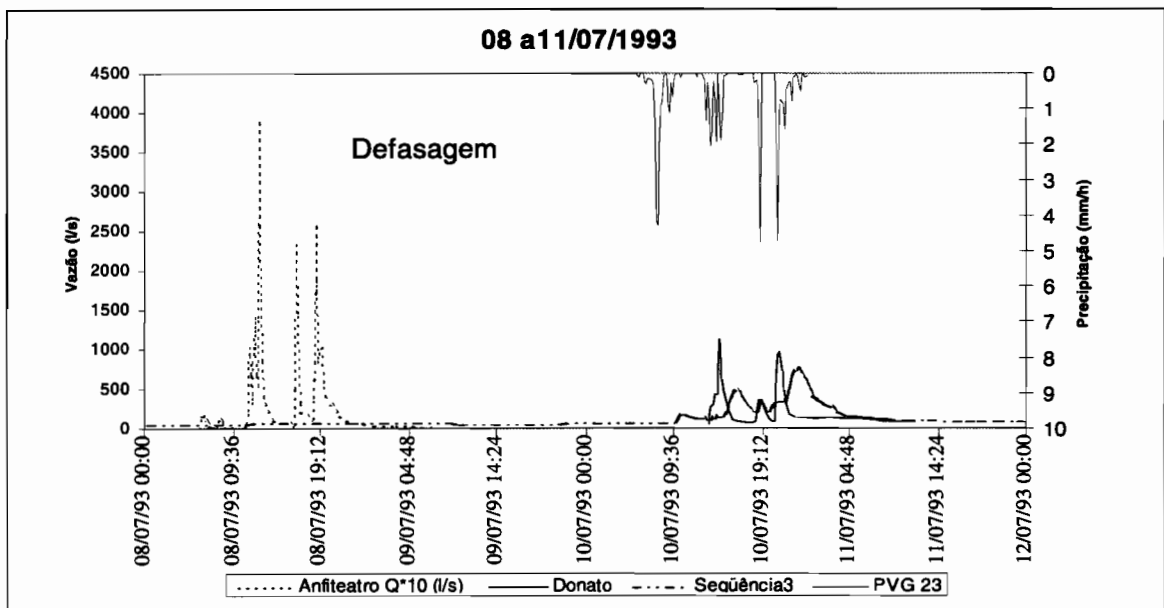
Figura 6.9 - Evento de 08 a 07/07/93
