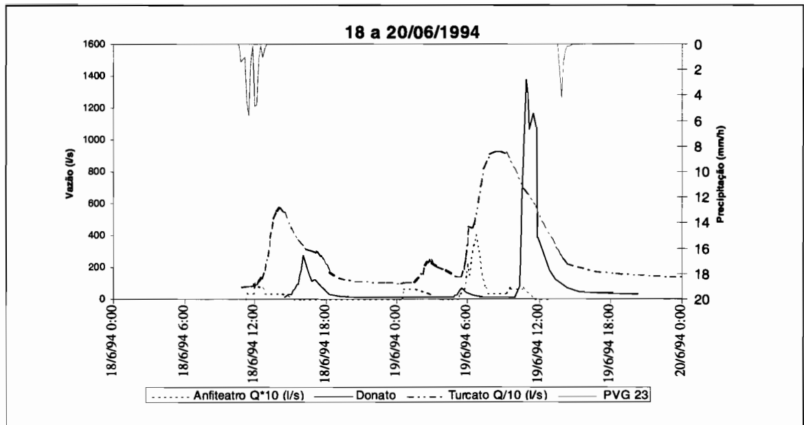
Figura 6.13 - Evento de 18 a 20/06/94
