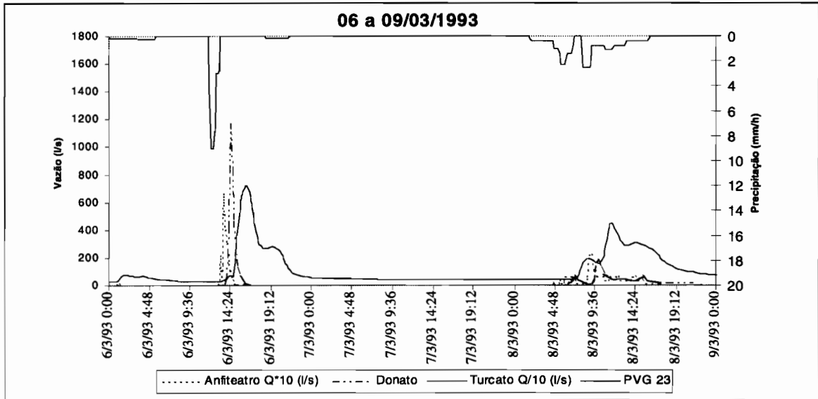
Figura 6.7 - Evento de 06 a 09/03/93
