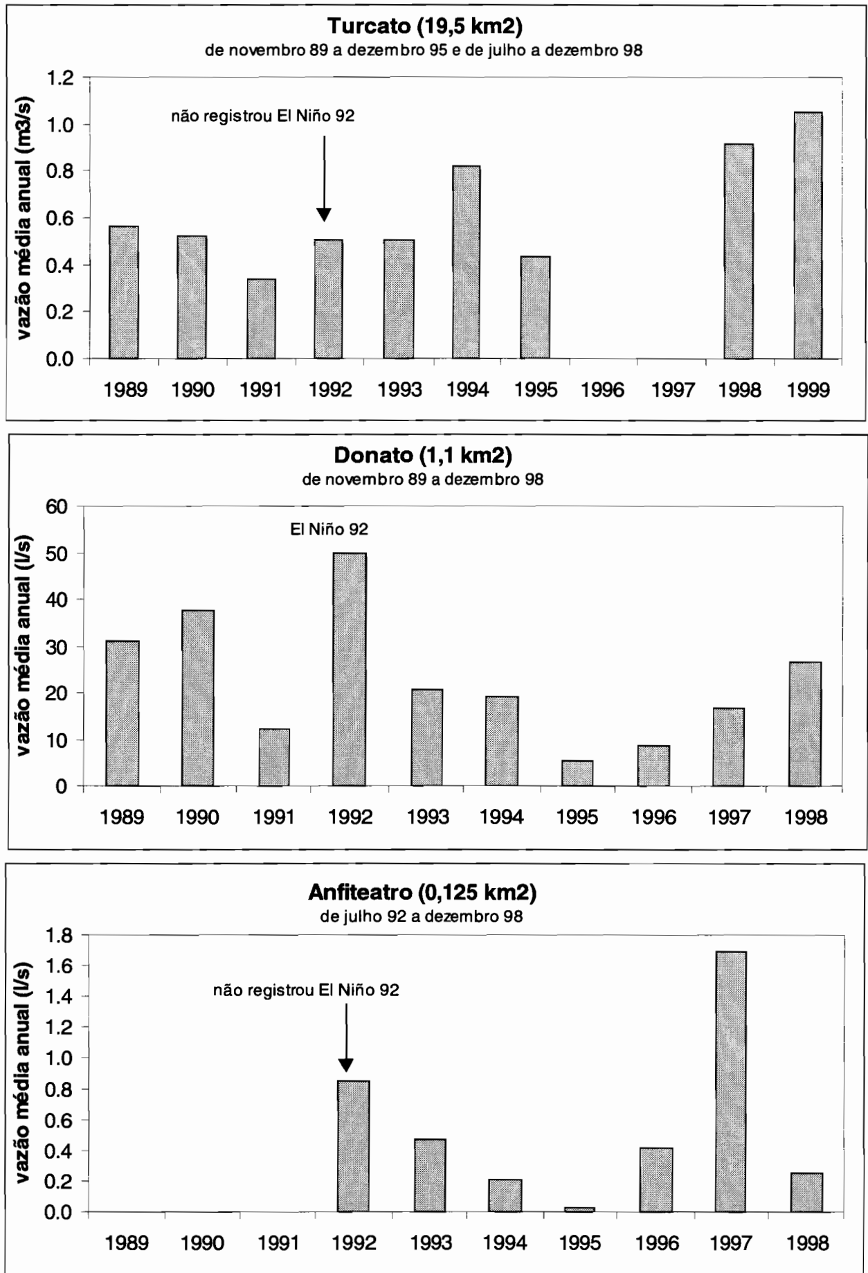
Figura 6.21 - Distribuição das vazões médias anuais das bacias Anfiteatro, Donato e Turcato
