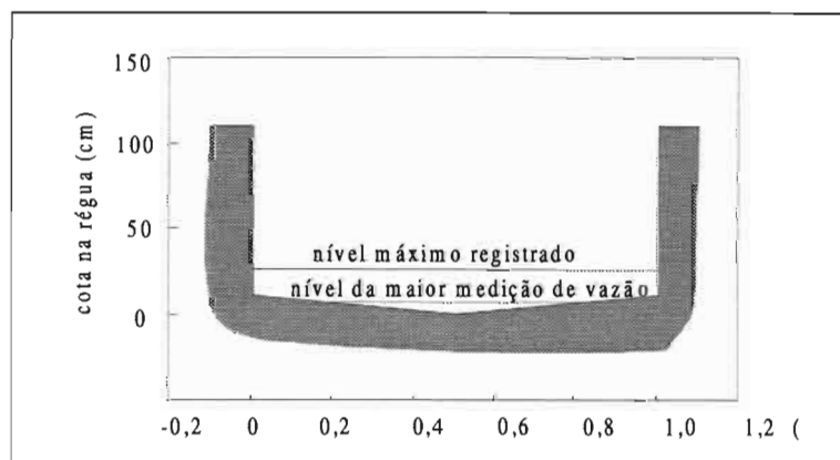
Figura 4.3 - Seção de medição na saída do Anfiteatro
