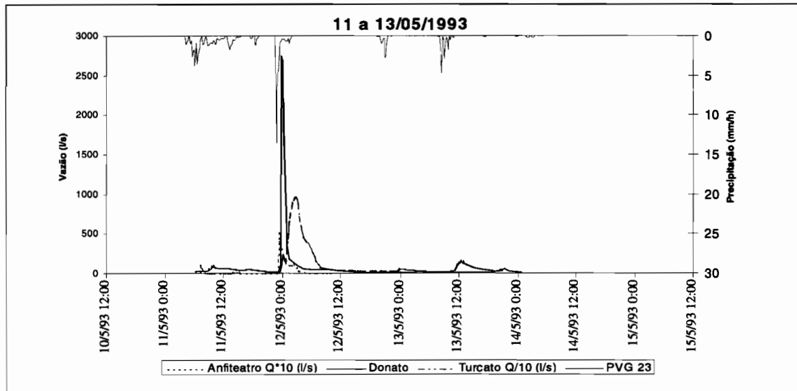
Figura 6.8 - Evento de 11 a 13/05/93
