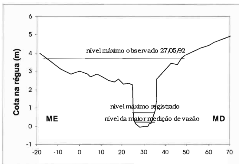
Figura 4.23 - Perfil transversal da seção de medição do Arroio Rincão
