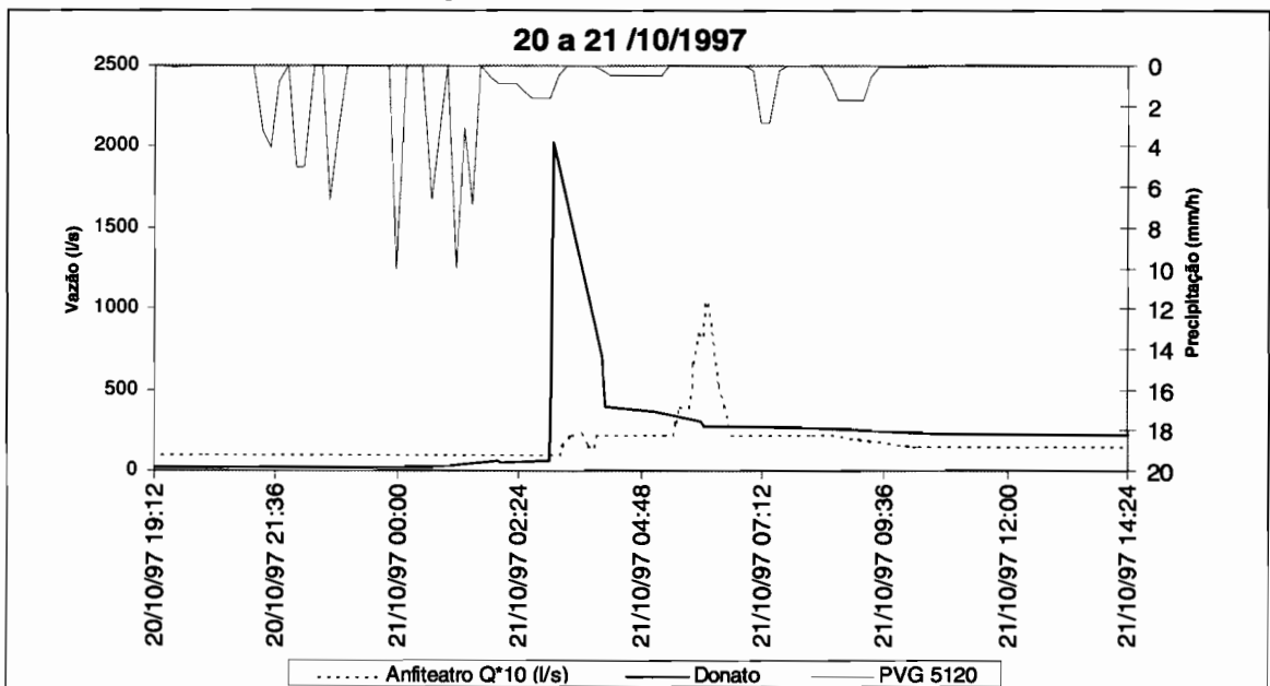
Figura 6.18 - Eventos de 20 a 21 /10/97
