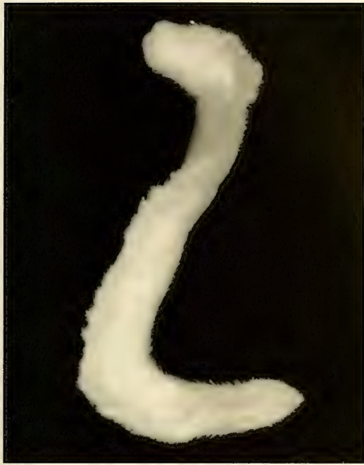
Fig. 2. Solenogastres: Eleutheromenia carinata , spec. nov. (9 mm; anterior end above).
