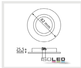
111063 | Einbaurahmen BRUSH, rund, Gu5,3, Alu gebürstet
