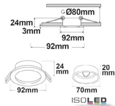
114007 | Einbaurahmen Kombi für GU10/MR16, schwarz + schwarz
