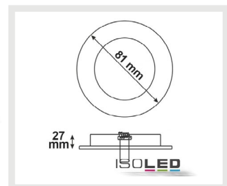
111048 | Einbaurahmen Ion, rund, Gu5,3, nickel satin
