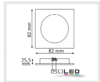
111062 | Einbaurahmen BRUSH, quadr., Gu5,3, Alu
