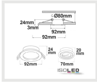
114015 | Einbaurahmen Kombi für GU10/MR16, Alu gebürstet + schwarz-gold
