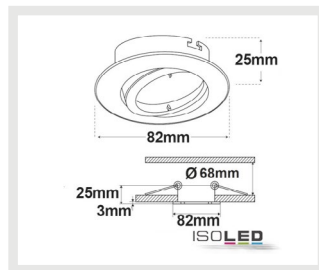
113713 | Einbaurahmen rund für GU10/MR16, Alu Nickel-Satin
