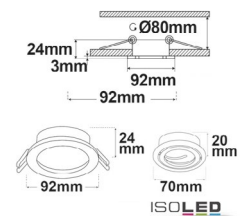
114010 | Einbaurahmen Kombi für GU10/MR16, weiß + schwarz-gold
