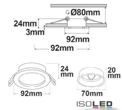
114008 | Einbaurahmen Kombi für GU10/MR16, schwarz + Alu weiß
