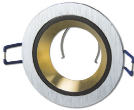
114015 | Einbaurahmen Kombi für GU10/MR16, Alu gebürstet + schwarz-gold
