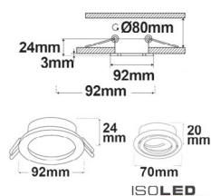
114011 | Einbaurahmen Kombi für GU10/MR16, weiß + weiß-silber
