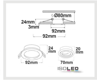
114016 | Einbaurahmen Kombi für GU10/MR16, Alu gebürstet + weiß-silber
