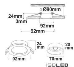
114012 | Einbaurahmen Kombi für GU10/MR16, weiß + schwarz
