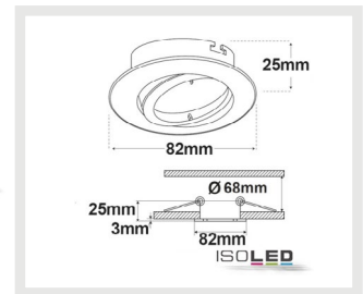
113712 | Einbaurahmen rund für GU10/MR16, Alu weiß
