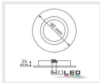
111047 | Einbaurahmen Ion, rund, Gu5,3, weiß
