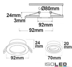
114009 | Einbaurahmen Kombi für GU10/MR16, schwarz + Alu gebürstet
