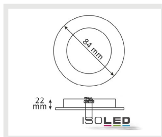
111049 | Einbaurahmen Ion, rund, Gu5,3, chrom
