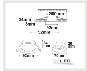
114018 | Einbaurahmen Kombi für GU10/MR16, Alu gebürstet + Alu weiß
