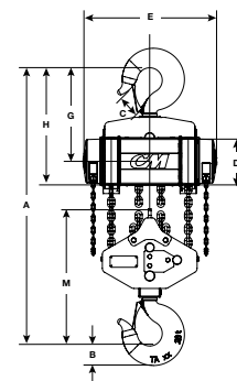
15 & 20 TON
