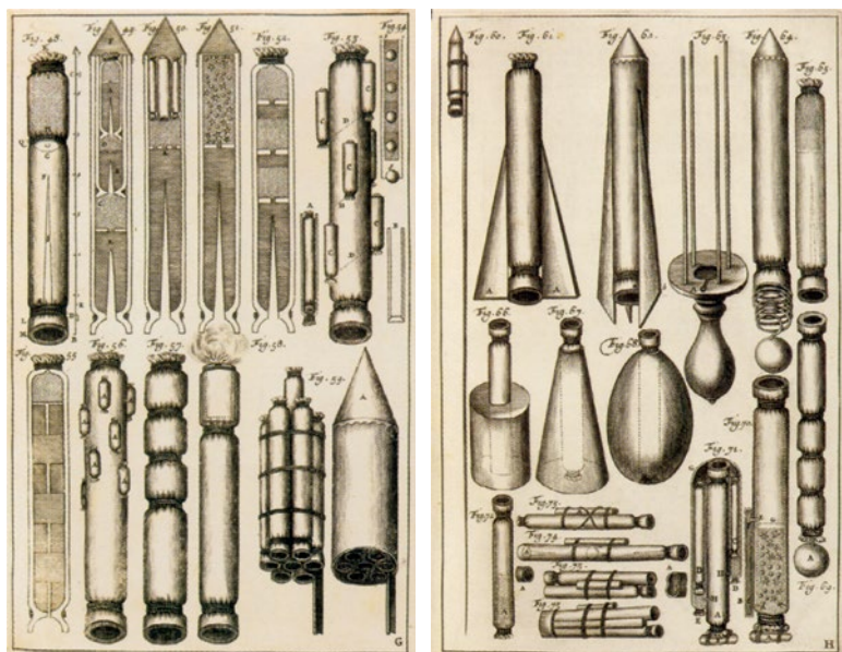
K. Semenavičiaus raketų brėžiniai. Amsterdamas, 1650 m.
