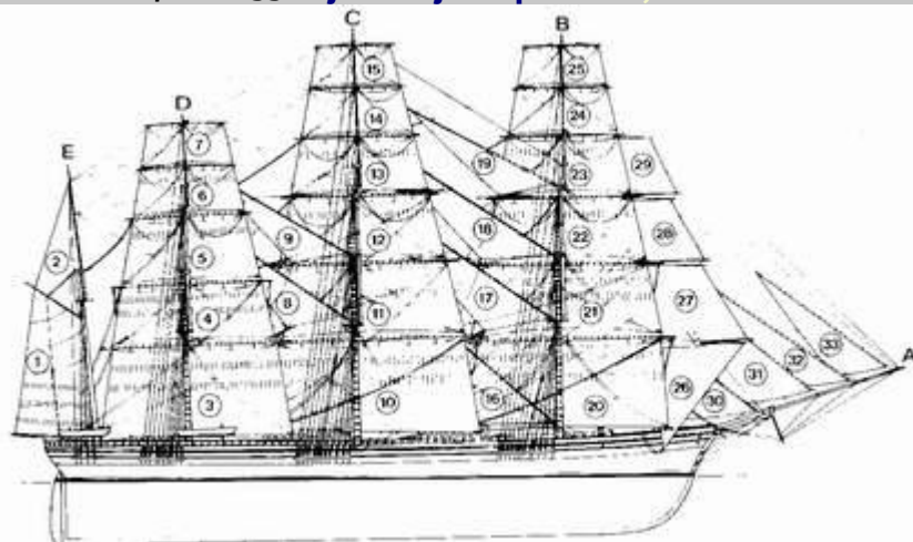
{1. šturnjača ili krmena sošnjača; 2. vrška; 3. stražnja debljača; 4. stražnja donja košnjača; 5. stražnja gornja košnjača; 6. stražnja sljemenjača; 7. stražnja vršnjača; 8. stražnja letka; 9. stražnja letkica; 10. glavna debljača; 11. glavna donja košnjača; 12. glavna gornja košnjača; 13. glavna donja sljemenjača; 14. glavna gornja sljemenjača; 15. glavna vrhovnjača; 16. glavna letnjača; 17. glavna letka; 18. glavna letkica; 19. glavna gornja letkica; 20. prednja debljača; 21. prednja donja košnjača; 22. prednja gornja košnjača; 23. prednja donja sljemenjača; 24. prednja gornja sljemenjača; 25. prednja vrhovnjača; 26. debleno pršno jedro (pršnjača, boneta); 27. donja košna pršnjača; 28. gornja košna pršnjača; 29. donja sljemena pršnjača; 30. letnjača; 31. prečnjača; 32. prečka; 33. prečkica.}
