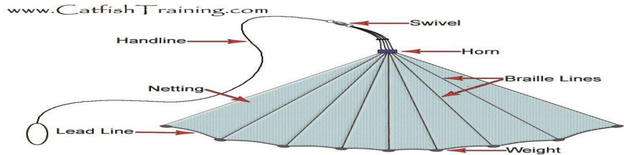
Fig. 42: Cast net
