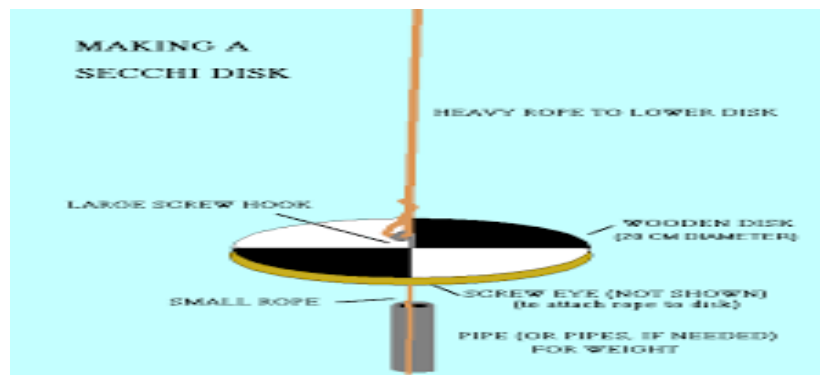
Fig.5: Secchi disk
