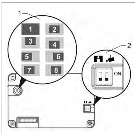
Abb. 24: Einstellung Kameramodul 180°
