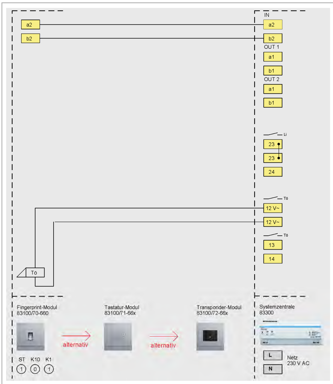
Abb. 39: Eine Außenstation mit Zutrittskontrolle
