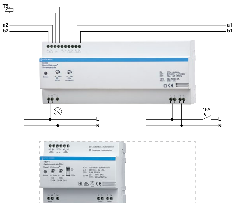
Direkter Türöffneranschluss
