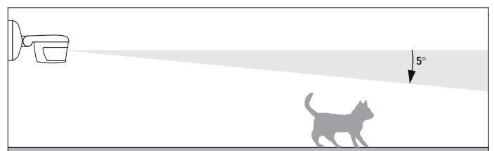
Günstig für die Außenüberwachung: Bei einer Anbringungshöhe von 1,5 m mit horizontaler Ausrichtung werden Kleintiere nicht erfasst
