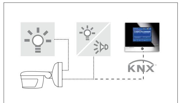
Ein zusätzlicher Schaltausgang ermöglicht das Auslösen eines optischen oder akustischen Alarmsignals im Haus, sobald jemand die Sicherheitszone betritt
