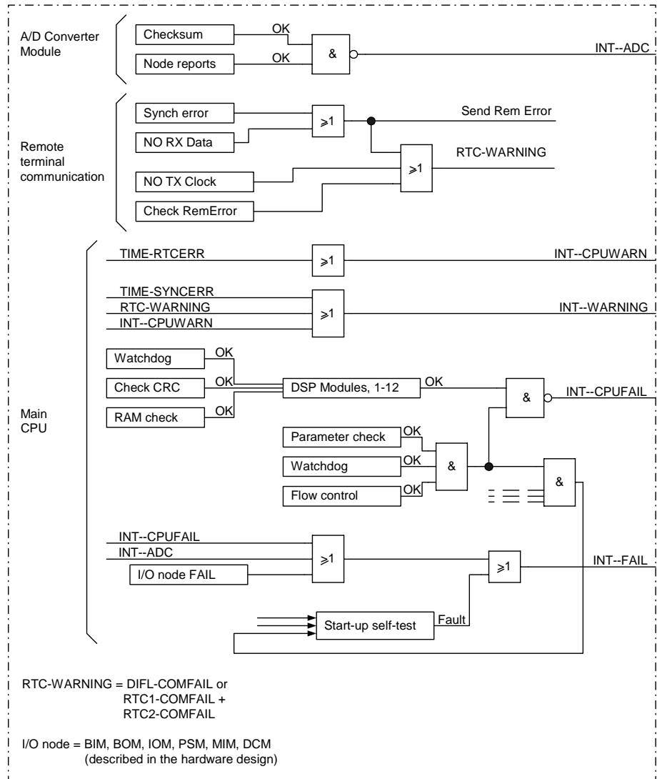
Abbildung 9: Software-Selbstüberwachung, INTerne Signale des Funktionsbausteins
