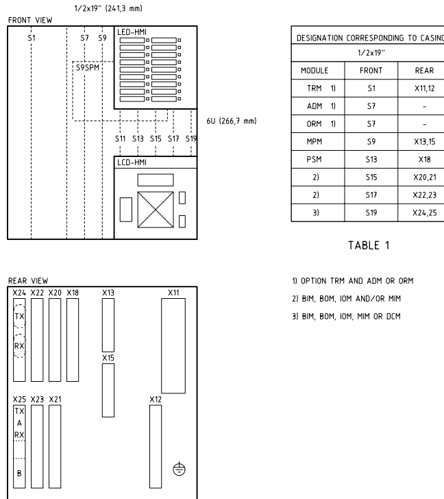
Abbildung 3: Bestückungsplan des 19-Zoll-Gehäuses mit halber Breite
