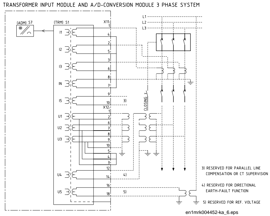
Abbildung 29: REB 551-C3, Meßwandlereingang-Modul und A/D-Wandler-Modul (dreiphasiges Netz)
