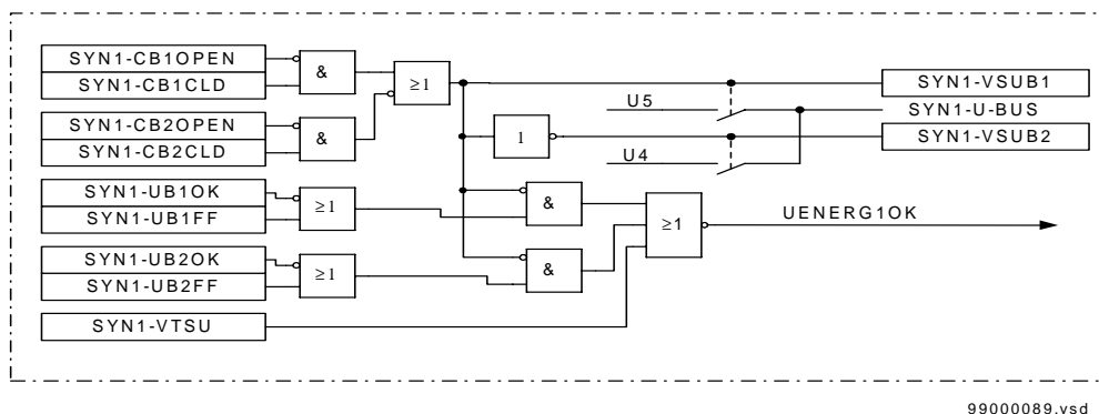
Abbildung 15: SYN, vereinfachte Spannungsauswahl-Logik in einer Konfiguration mit Doppelsammelschienen und individuellem Leistungsschalter
