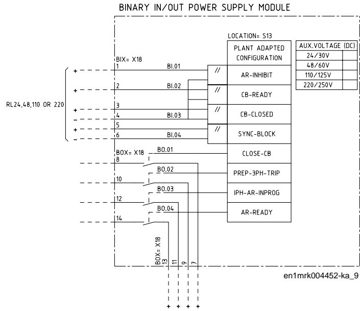
Abbildung 32: REB 551-C3, Spannungsversorgungsmodul mit binären Ein-/Ausgängen
