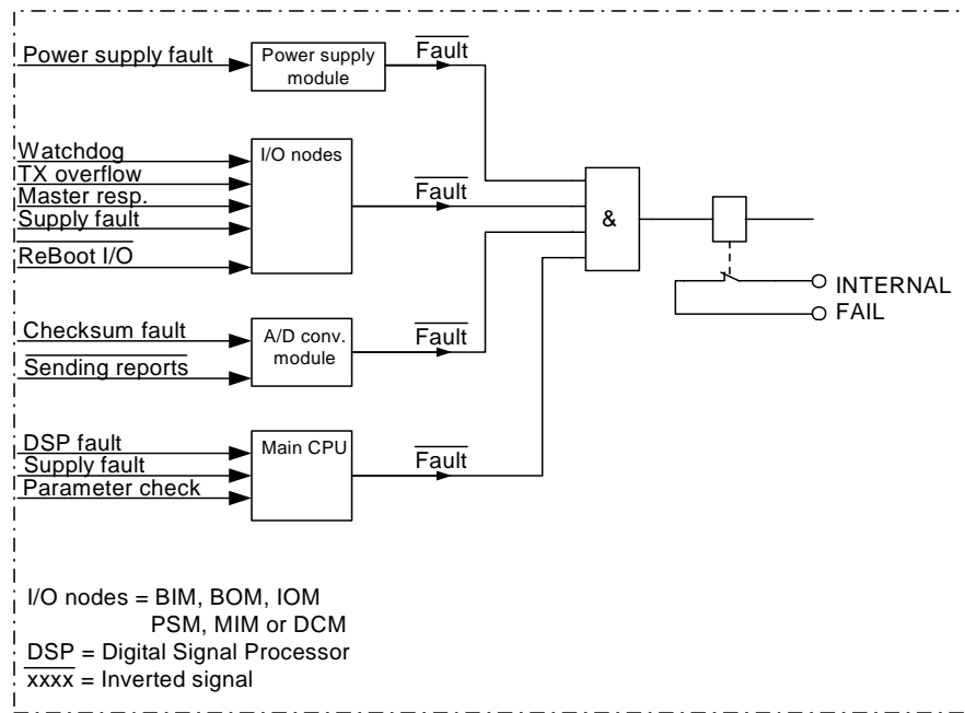
Abbildung 8: Hardware-Selbstüberwachung, potentialfreier Alarmkontakt.
