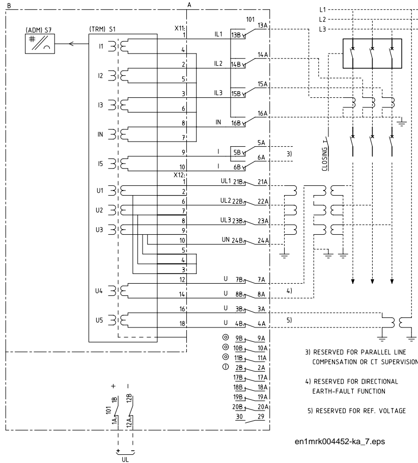
Abbildung 30: REB 551-C3, Meßwandlereingang-Modul und A/D-Wandler-Modul (dreiphasiges Netz) mit RTXP 24, interne Erdung
