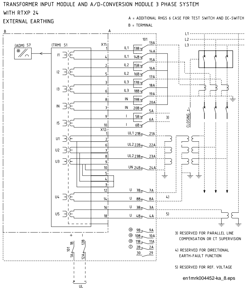
Abbildung 31: REB 551-C3, Meßwandlereingang-Modul und A/D-Wandler-Modul (dreiphasiges Netz) mit RTXP 24, externe Erdung
