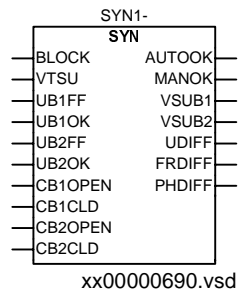
Abbildung 13: Funktionsbaustein für Einzel-Leistungsschalter
