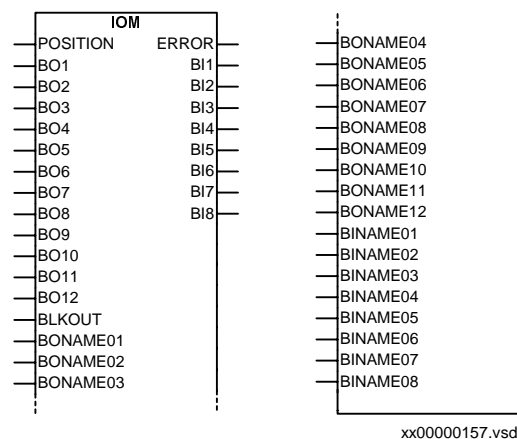
Abbildung 24: E/A-Modul
