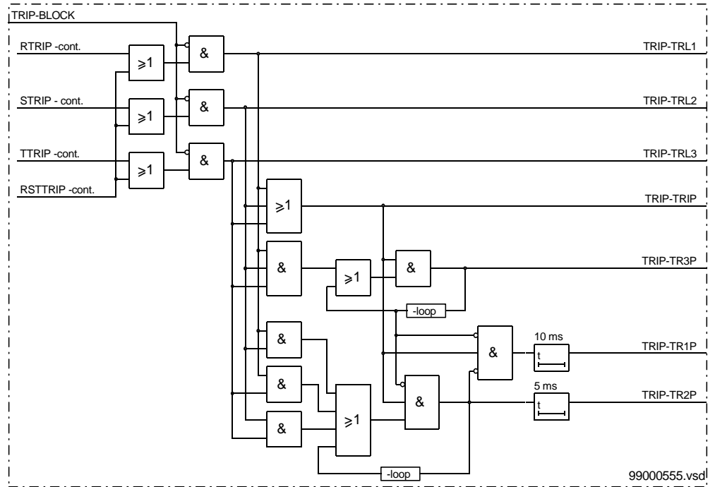
Abbildung 22: End-Auslöseschaltungen
