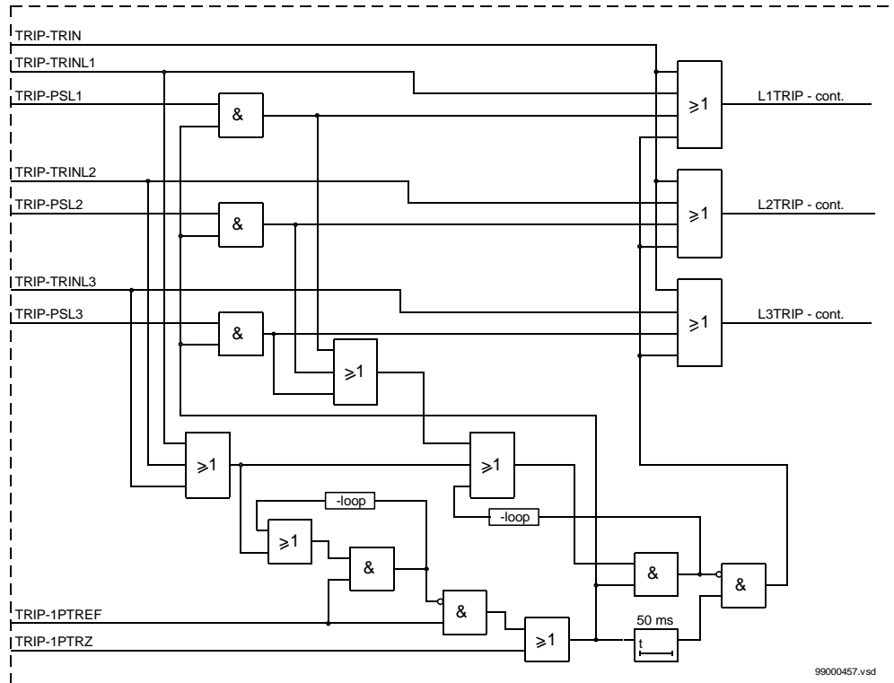
Abbildung 19: Phasengetrennte Logik vorn
