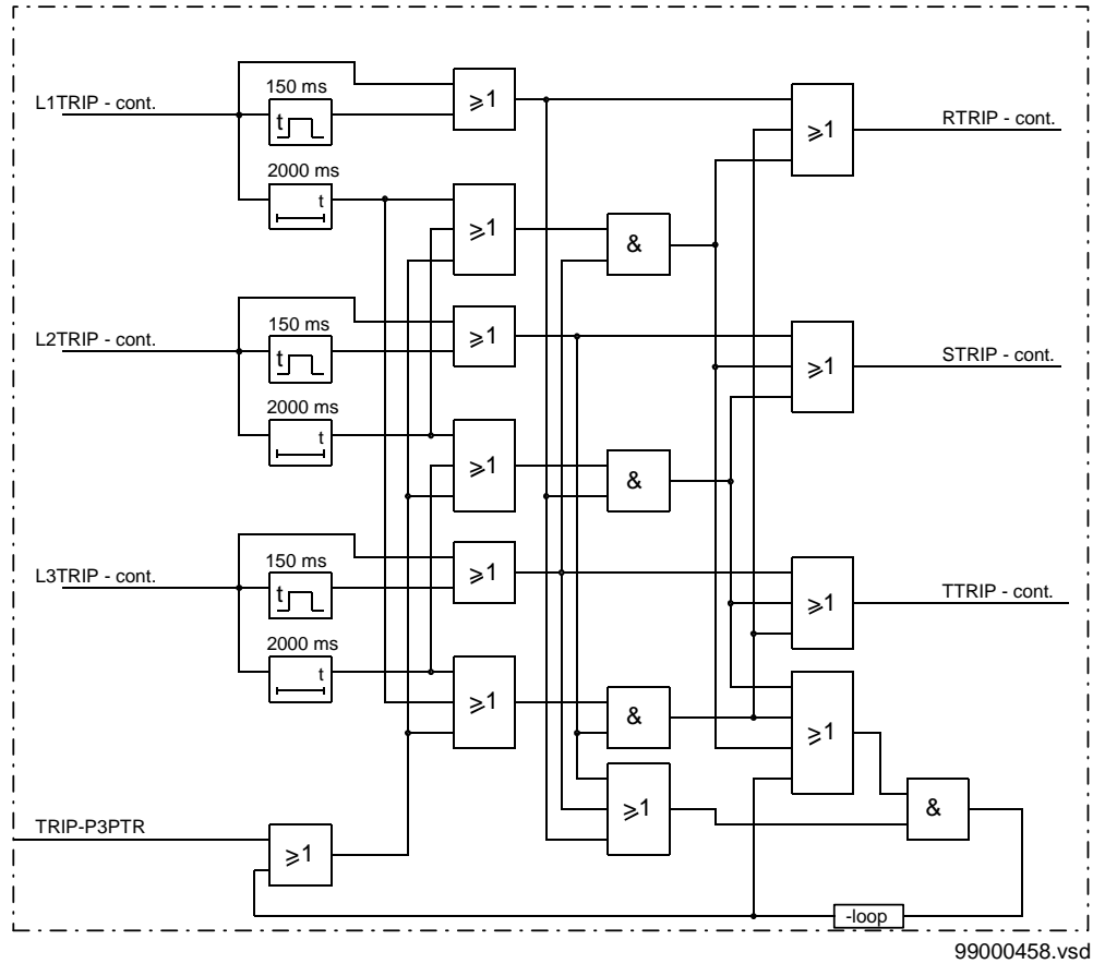
Abbildung 20: Zusatzlogik für die ein-/dreiphasige Betriebsart
