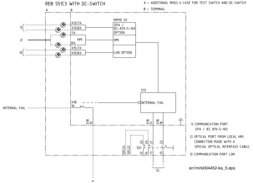
Abbildung 28: REB 551-C3 mit Gleichspannungsschalter
