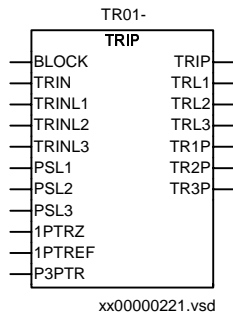
Abbildung 17: Funktionsbaustein TR: Logik für ein-, zwei- und/oder dreipolige Auslösung
