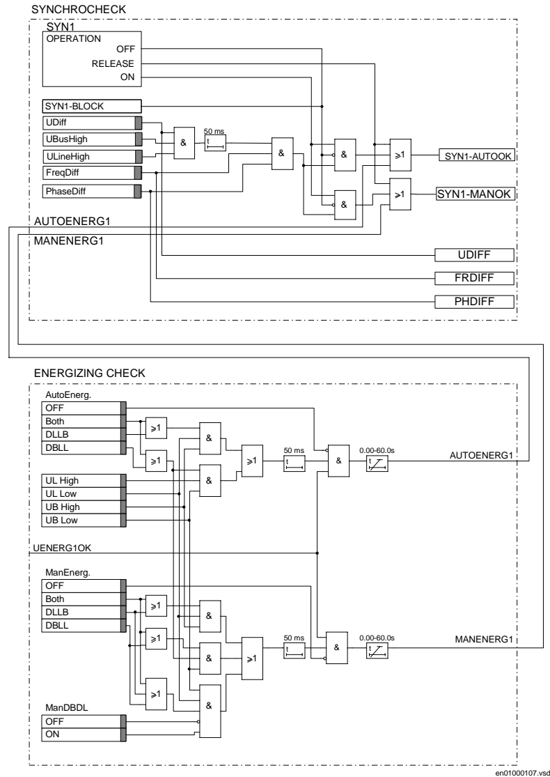
Abbildung 14: SYN, vereinfachtes Logikdiagramm; Synchronvergleich und Zuschaltkontrolle. Das interne Signal UENERG1OK bezieht sich auf die Spannungsauswahl-Logik
