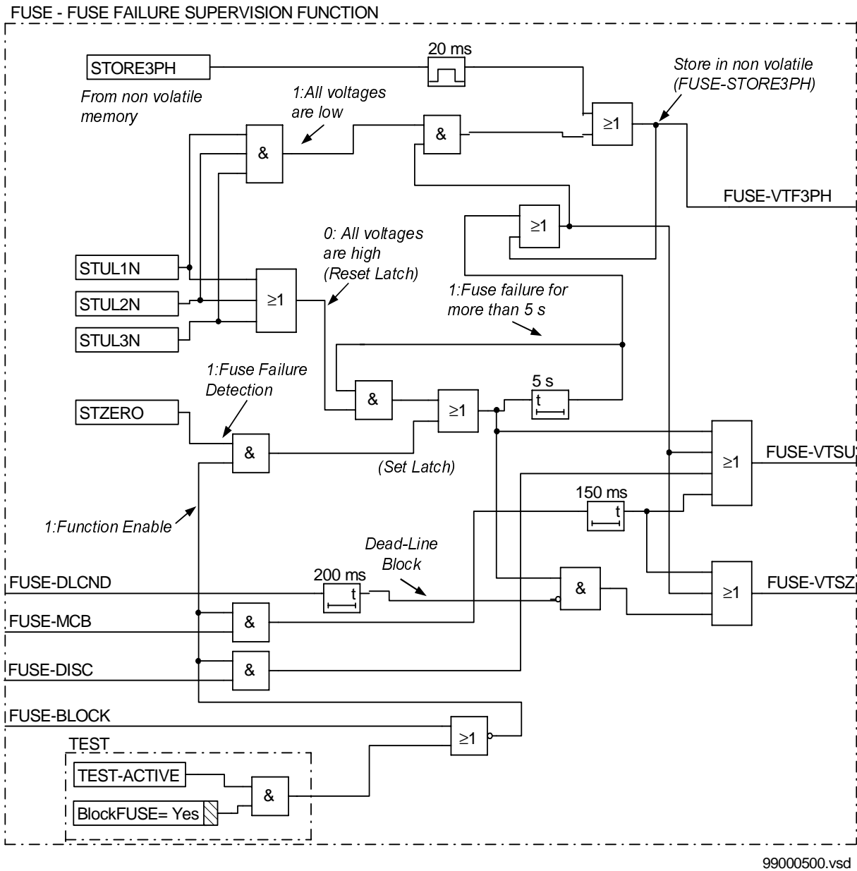
Abbildung 12: Vereinfachtes Logikdiagramm für die Funktion Sicherungsüberwachung, Nullsystem
