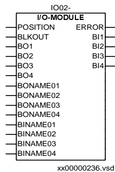
Abbildung 25: Binäre Ein-/Ausgänge am Spannungsversorgungsmodul PSM
