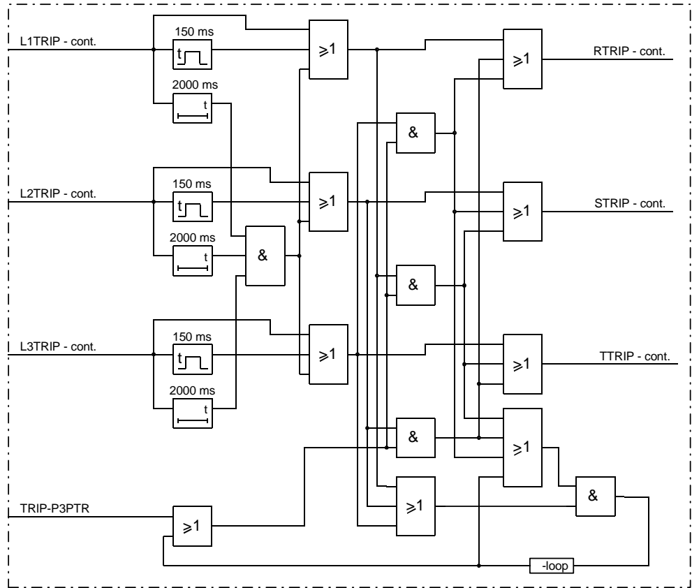
Abbildung 21: Zusatzlogik für die ein-/zwei-/dreiphasige Betriebsart
