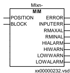
Abbildung 23: Ein MIM-Modul (mA-Meßeingangs-Modul) besitzt sechs Eingangskanäle. Jeder Kanal verfügt über einen Funktionsbaustein, M I_x n-, wobei x=(1-6) die Nummer des MIM-Moduls angibt und n=(1-6) der Nummer des Kanals entspricht.
