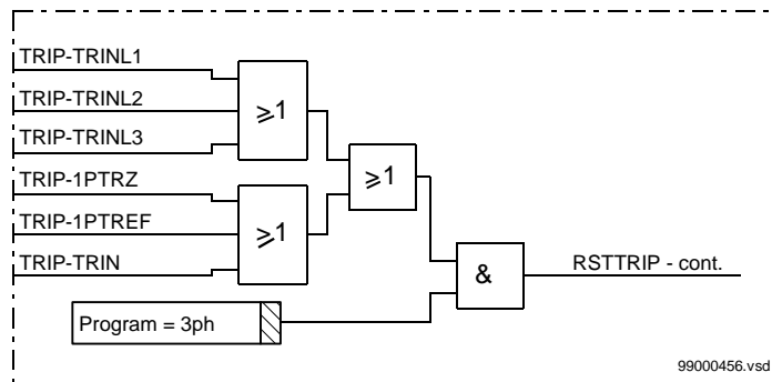
Abbildung 18: Dreiphasige Logik vorn – vereinfachtes Logikdiagramm
