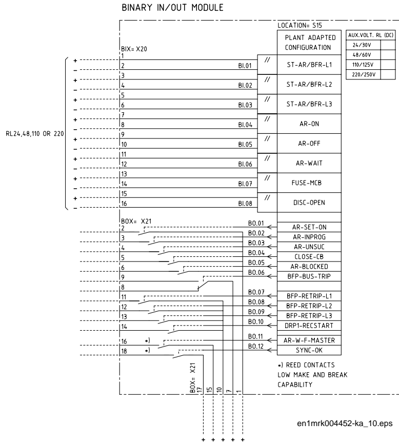
Abbildung 33: REB 551-C3, Binär-Ein-/Ausgang-Modul
