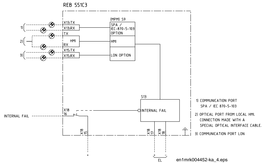
Abbildung 27: REB 551-C3
