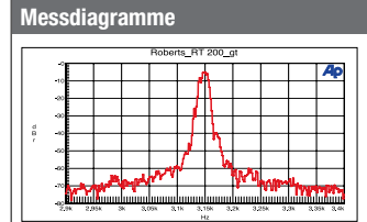
Gleichlauffton-Spektrum Etwas aufgeweitete Spitze, aber recht schnell abfallend ohne nennenswerte Seitenbänder
