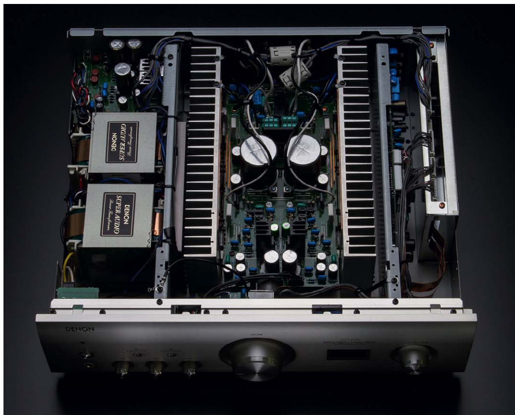
Bei dem in insgesamt sechs Funktionsblöcke aufgeteilten Vollverstärker sitzt der DAC in einer abgeschirmten Sektion. USB-Abteilung und koaxiale Eingänge wurden auch elektrisch isoliert, hier blockieren Übertrager hochfrequenten Rauschen und andere Störungen, die vom Rechner herrühren können.
