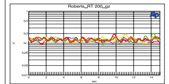
Gleichlaufschwankungen vs. Zeit Durchweg gleichmäßige Abweichungen ohne Regelmäßigkeiten auf gutem Niveau
