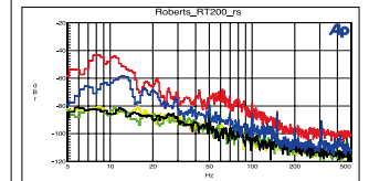
Rumpel-Spektrum Erstaunlich hoher Störabstand mit Platte, mit Koppler hervorragend gerade im Hörbereich
