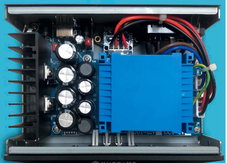
Rechts: Das Netzteil LPS-205 ist mit Trafo und Spannungsreglern aufgebaut und kann auch den Netzwerk-Switch SW-8 versorgen. Der erlaubt den Anschluss von 8 Teilnehmern.
