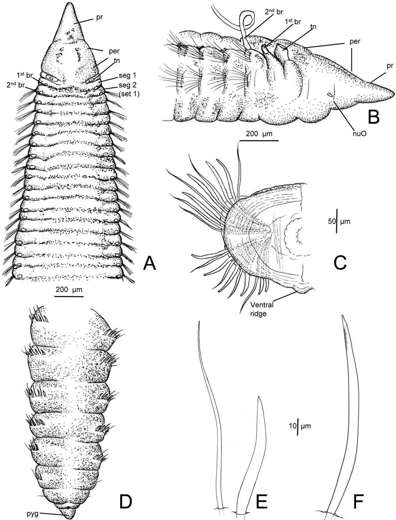
FIGURE 3. Chaetozone pigmentata n. sp. Paratypes (USNM 51221): A, anterior end, dorsal view; B, anterior end, right lateral view; C, far posterior parapodium, anterior view; D, posterior end, dorsal view; E, neuropodial acicular spine and capillary from far posterior segment; F, notopodial acicular spine from far posterior segment. (All paratypes, USNM 51221).
