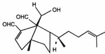
(6R)-6-hydroxydichotoma-3,14-diene-1,17-dial
