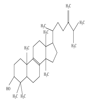
Euphorbol
