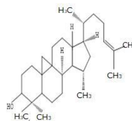
Cycloartenol
