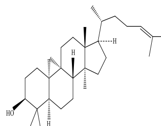
Nerifolione
