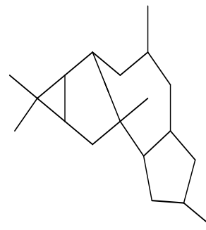
Ingenane (1&amp;2)
