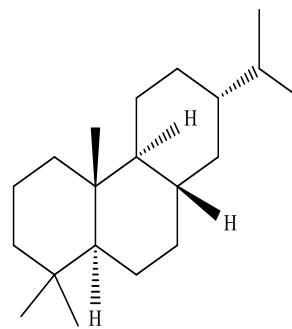
Abietane
