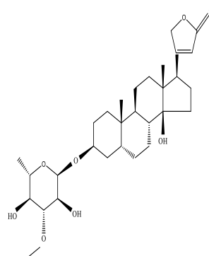
Neriifolin-S
