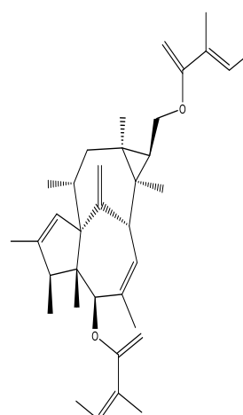
Euphorneroid A
