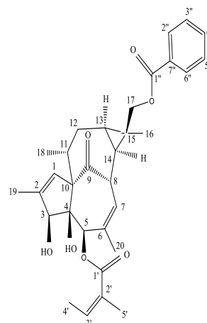
Eurifoloid E
