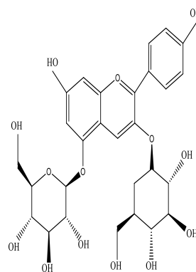
Pelargonin-3,5-diglucoside
