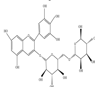
Tulipanin
