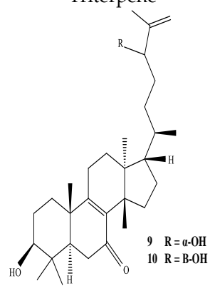
Triterpenes
