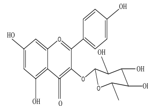
Afzelin
