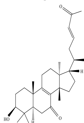
Triterpenes
