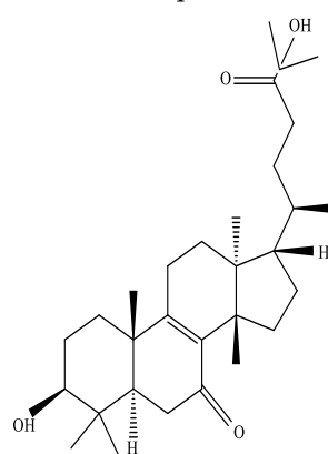
Neritriterpenols E
