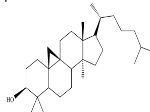
Cycloartenol
