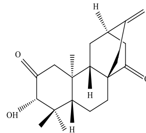
Ent-3S-hydroxyatis-16(17)-en-1,14-dione
