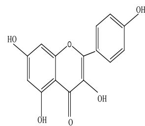
Kaempferol
