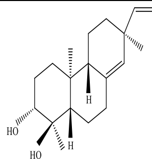
Eupneria J
