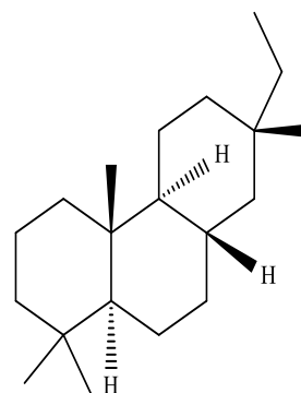
Isopimarane
