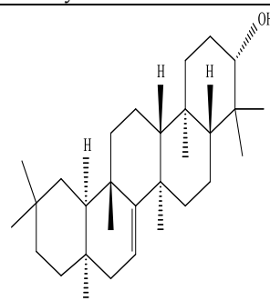
Taraxerol
