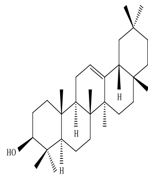
\beta -Amyrin
