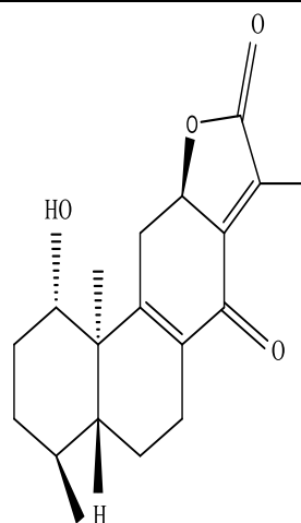
Eupnerias F
