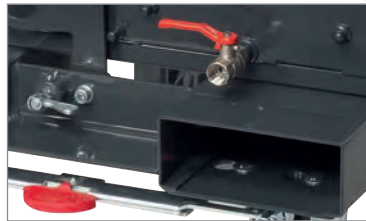
Ablasshahn mit Sieb zum Trennen von Flüssigkeiten und Feststoffen. TOTALSTOP-Zentralbremssystem.
