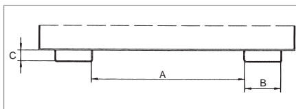
Einfahrtaschen-Maße: A: 465 mm B: 170 mm C: 55 mm
