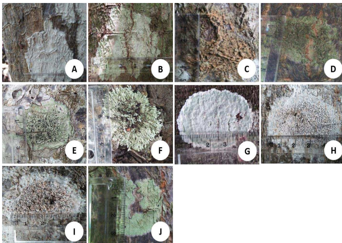
Gambar 1. Jenis-jenis lichen di Hutan Mangrove Desa Tomoli: A. Asp icilia calcarea (L.) Mudd, B. Asp icilia sp., C. Pyrenula dermatodes (Borrer) Schaer, D. Pyrenula santensis (Nyl) Mull. Arg, E. Pyrenula sp., F. Flavoparmelia caperata (L.) Hale, G. Cryptothecia striata (Ehrenb) G. Thor, H. Phaeographis sp., I. Graphis scripta (L.) Ach, dan J. Verrucaria sp.
