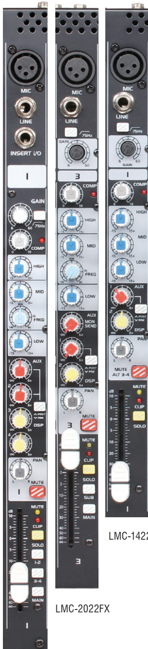
LMC-2624FX
