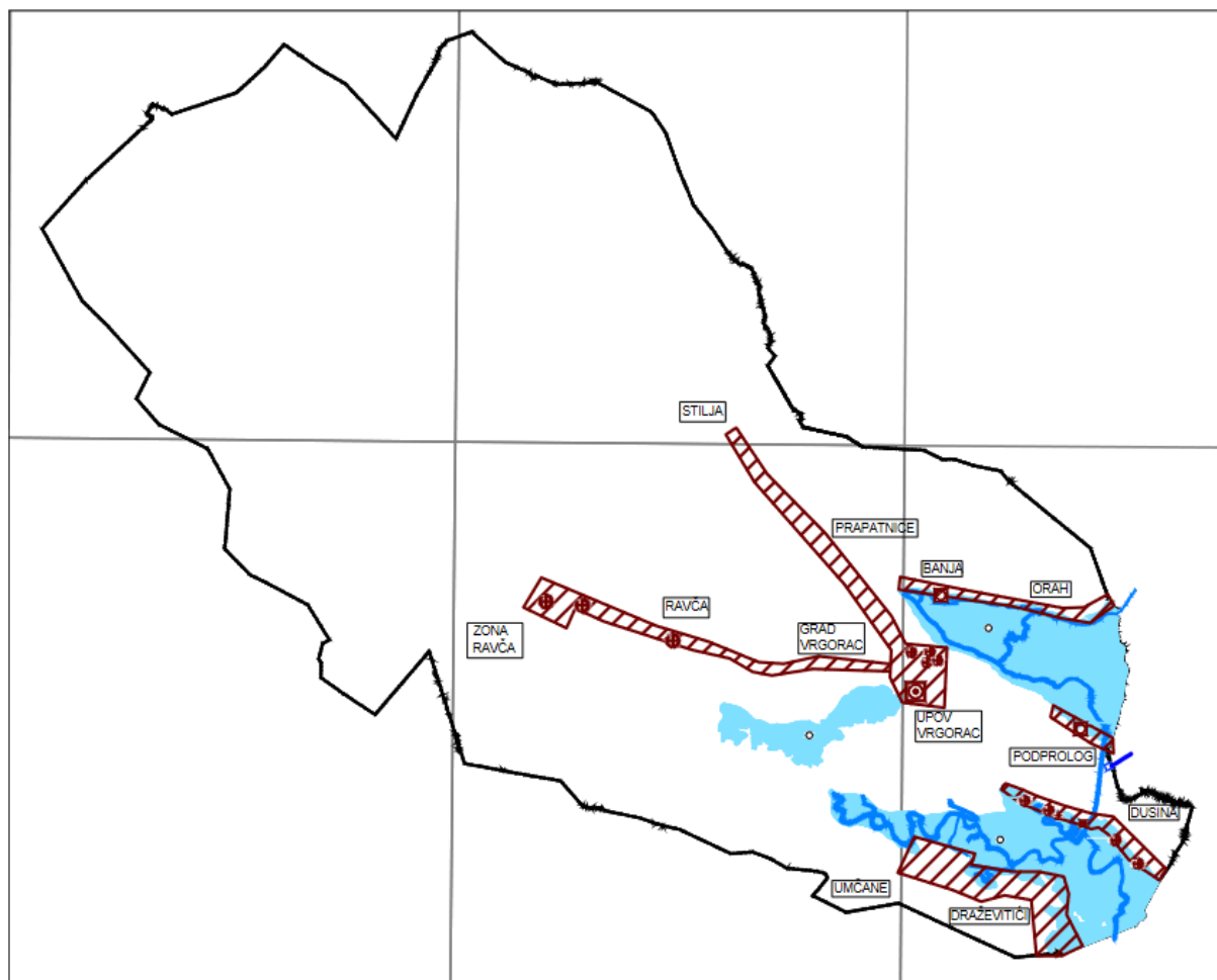
Slika 14. Plan izgradnje sustava odvodnje u narednom razdoblju trajanja PUR-a
