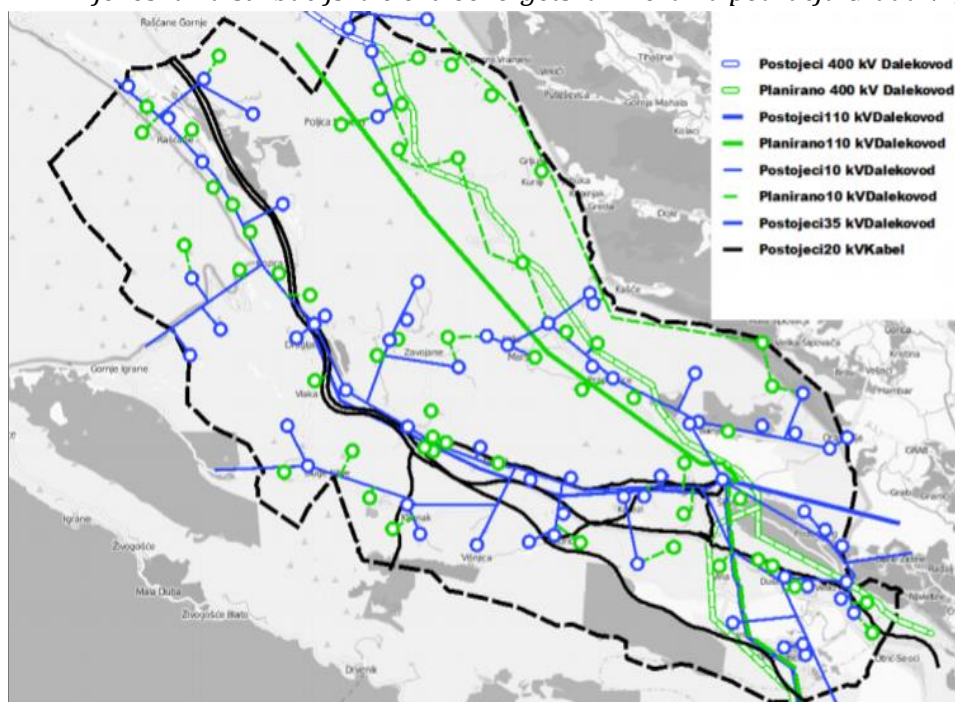
Slika 15. Prijenosna i distribucijska elektroenergetska mreža na području Grada Vrgorca
