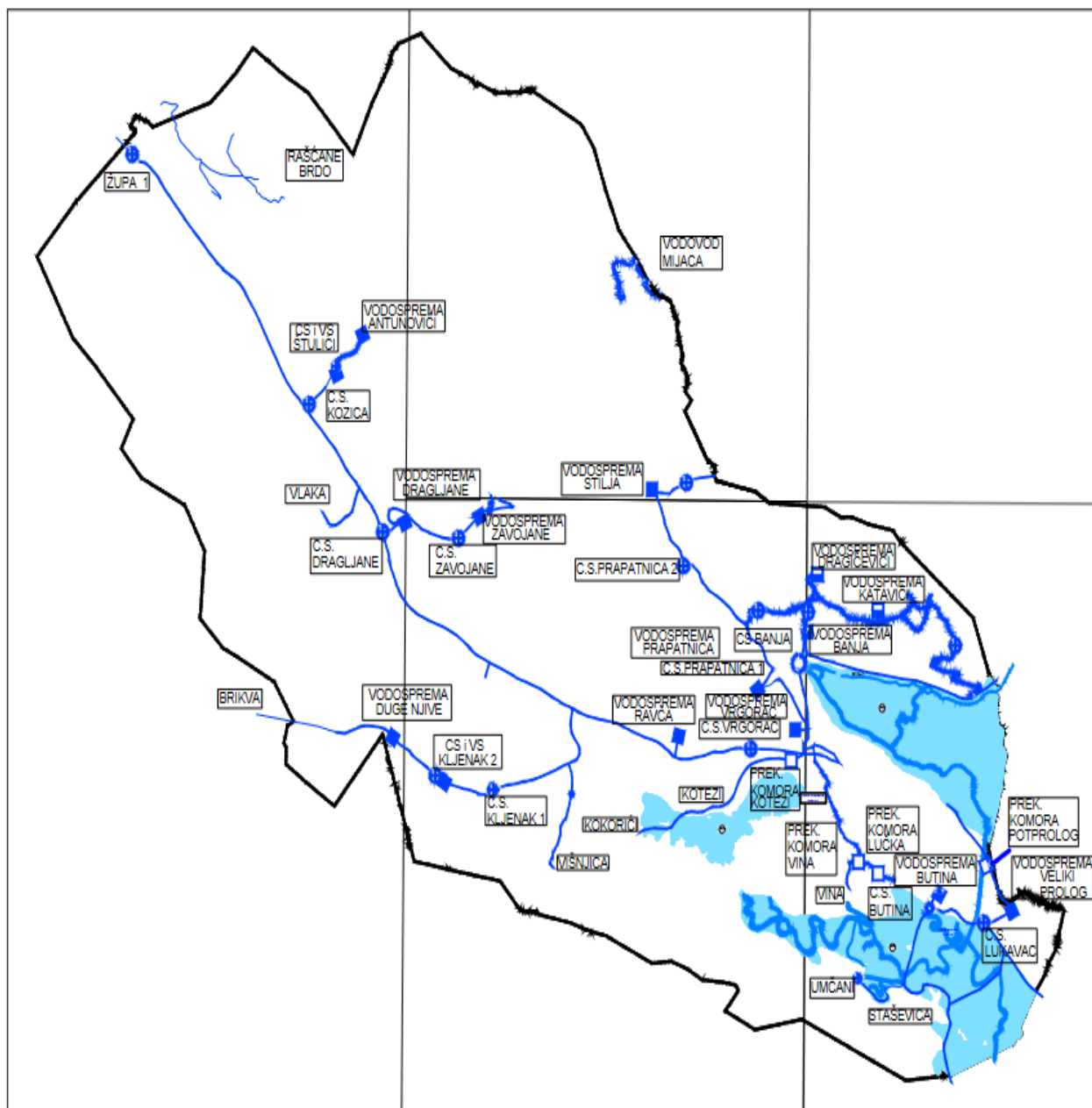
Slika 12. Plan izgradnje vodoopskrbnog sustava u narednom razdoblju trajanja PUR-a
