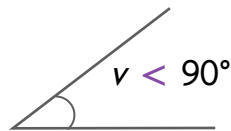
Spetsig vinkel
