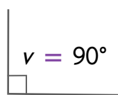
Rät vinkel
