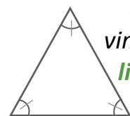
Liksidig triangel
