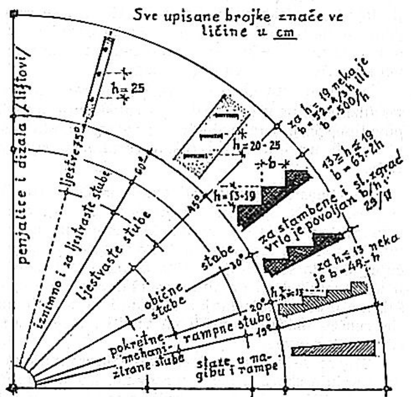
Sl. 920. Pregled primjene različitih uređaja za savladavanje visinskih razlika
