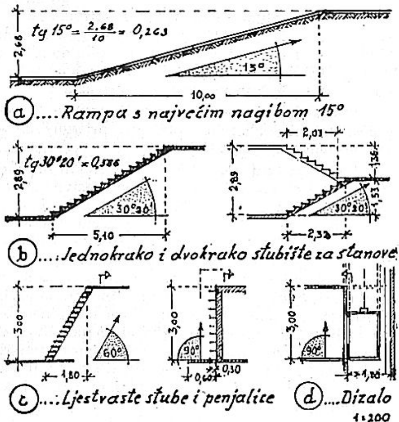
Sl. 919. Sheme četiriju osnovnih skupina građevinsko-tehničkih uređaja za uzlaženje i silaženje
