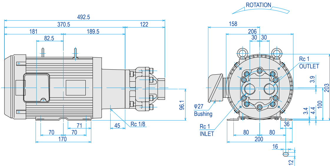
Model : TOP-3MF2200-N3**FAVB** IE3
