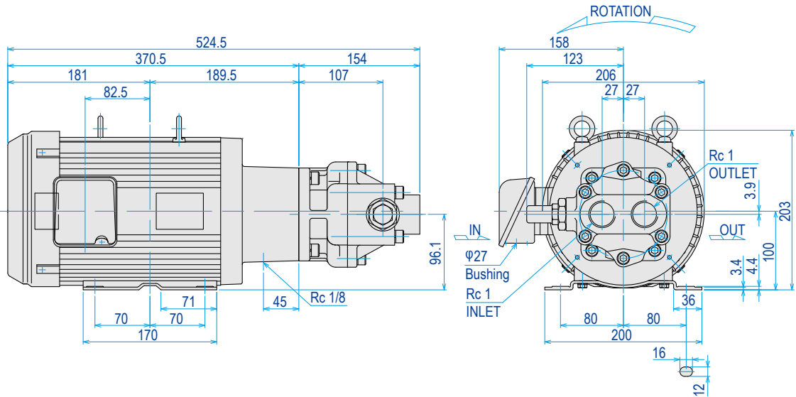
Model : TOP-3MF2200-N3**FB** IE3
