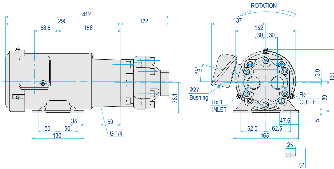
Model : TOP-3MF750-N3**FAVB-** IE3
