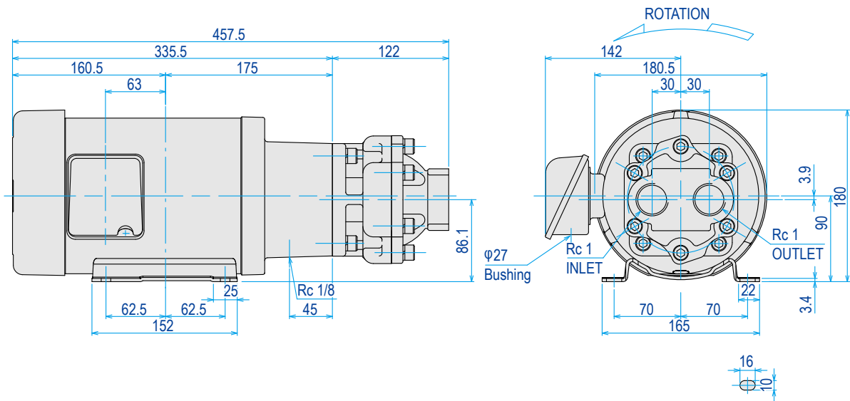
Model : TOP-3MF1500-N3**FAVB** IE3
