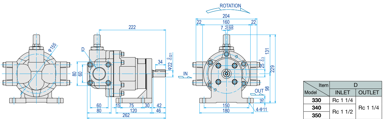
Model : TOP-3**VF-**
