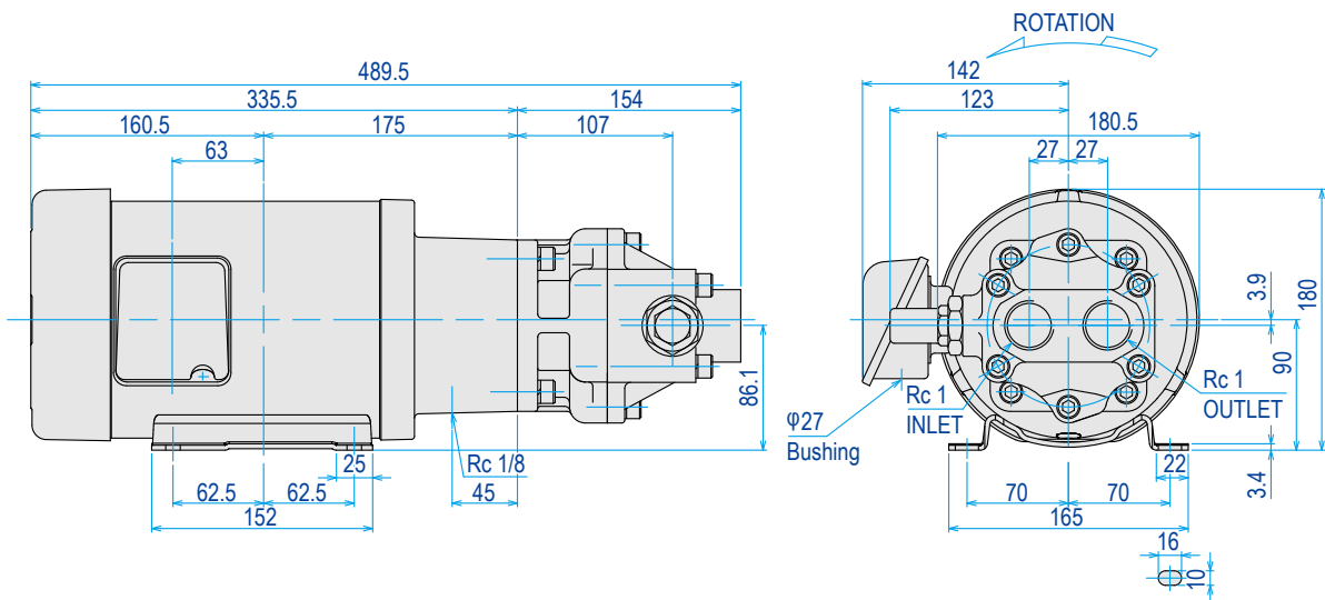
Model : TOP-3MF1500-N3**FB** IE3
