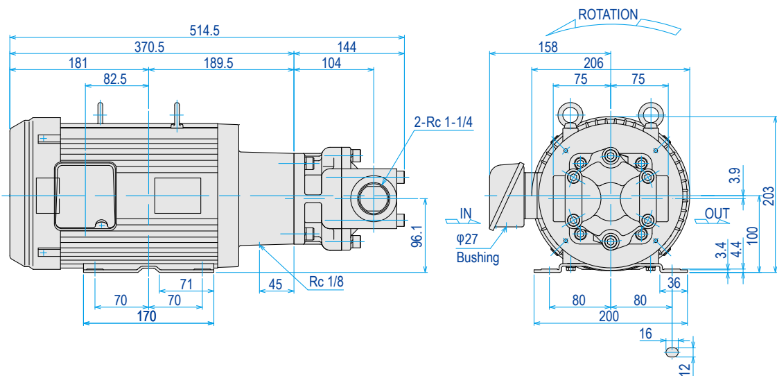
Model : TOP-3MF2200-N3**FB** IE3
