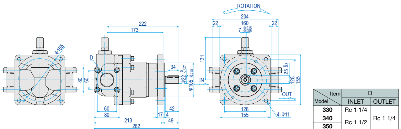
Model : TOP-3**VFVB-**
