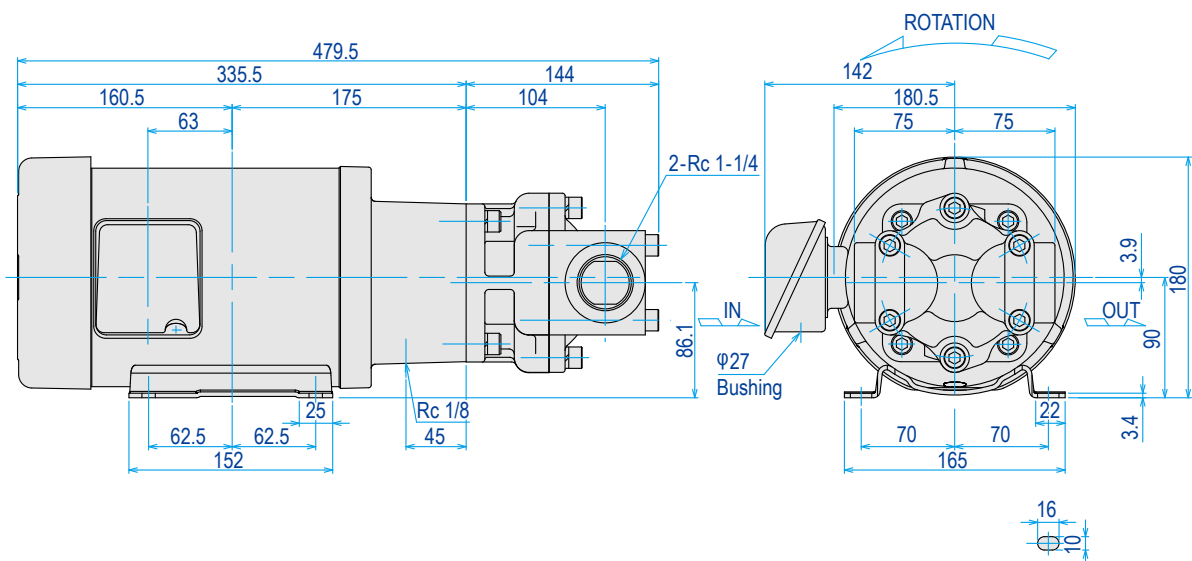
Model : TOP-3MF1500-N3**FB** IE3
