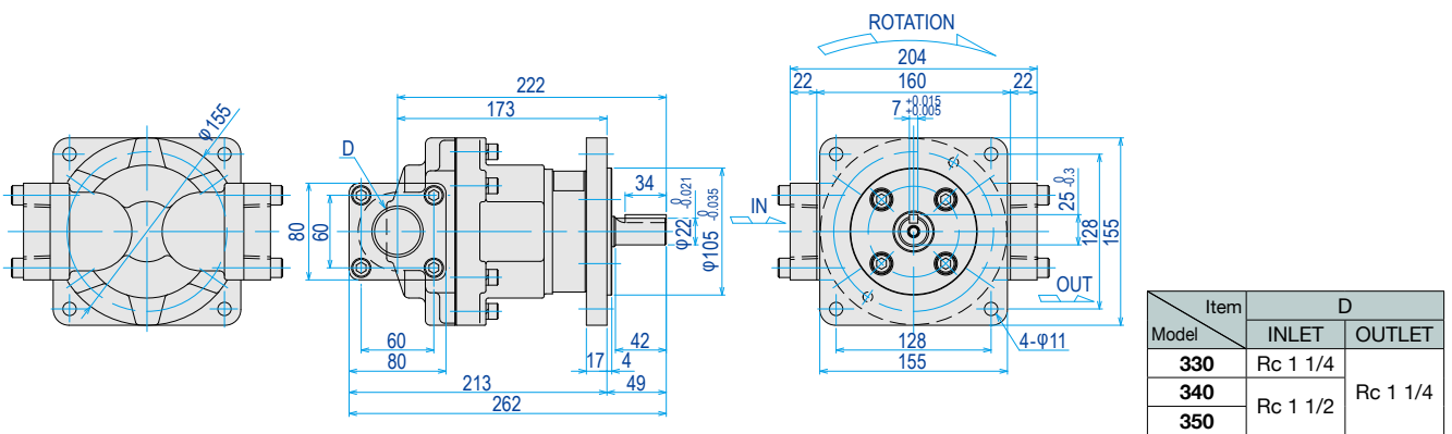
Model : TOP-3**VFVB-**
