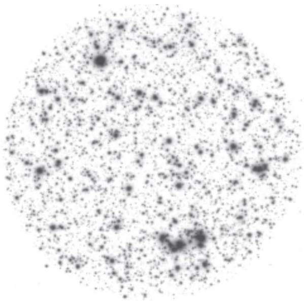
Figure XIII.8. Autoradiogram of an air filter sample taken from a nuclear power plant during maintenance ( http://www.stuk.fi/julkaisut_maaraykset/kirjasarja/fi_FI/kirjasarja2/ ). The diameter of the image is about 10 cm.
