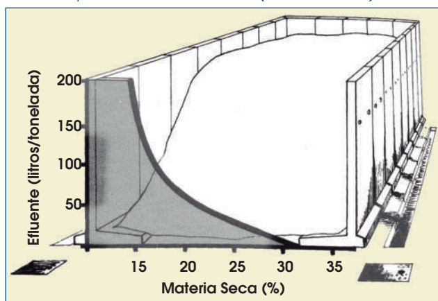
Figura 4. Efecto del porcentaje de MS del forraje en la producción de efluentes (Wilkinson, 2005)
