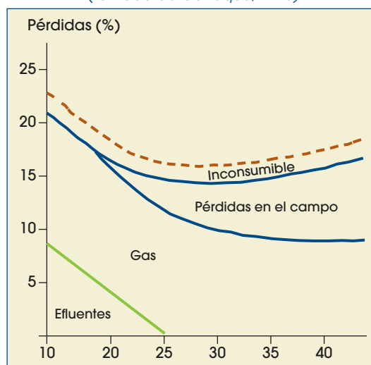
Figura 12. Pérdidas en ensilados de hierba según el contenido en MS en el momento de ensilar (tomado de Cañeque, 1998)
