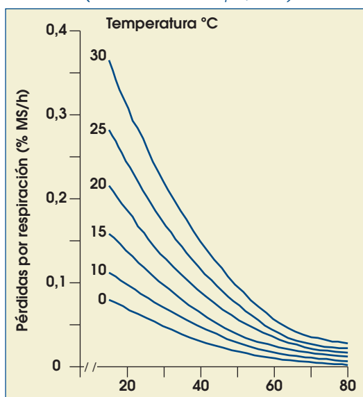
Figura 2. Pérdidas por respiración en el campo (tomado de Cañeque, 1998)
