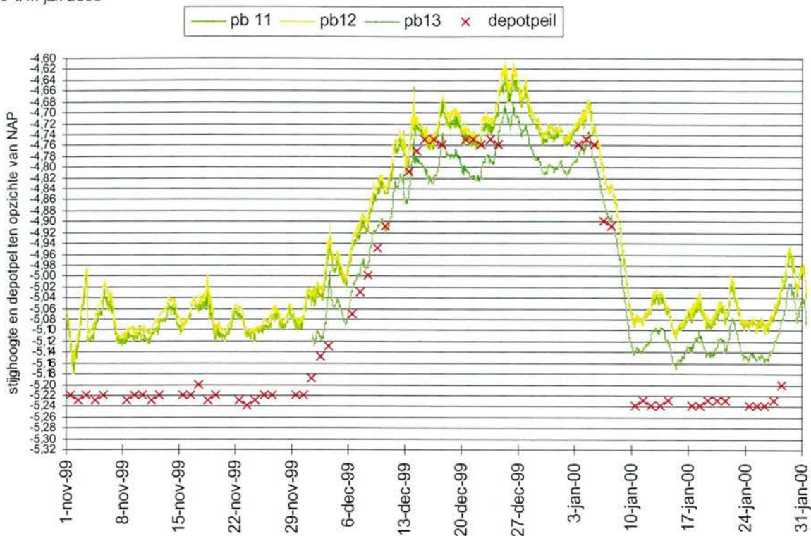
Figuur 27 Stijghoogte en depotpeil westkant depot dec 1999 en jan 2000
