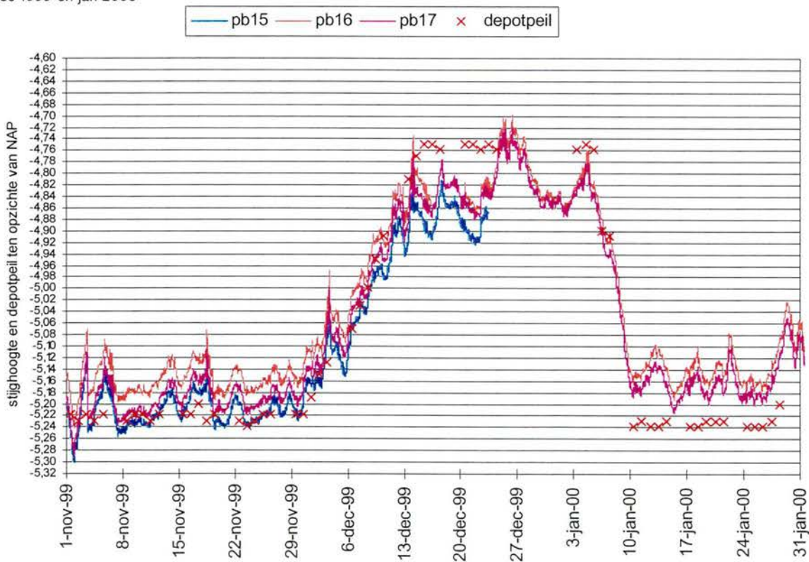
Figuur 27 Stijghoogte en depotpeil westkant depot dec 1999 en jan 2000
