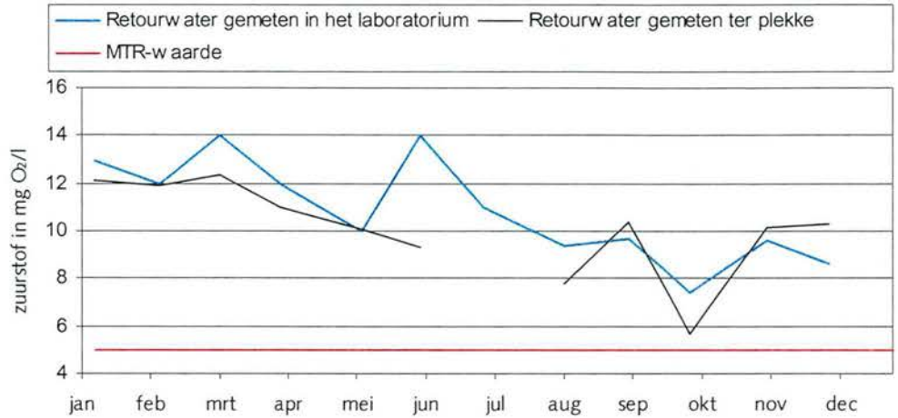
Figuur 5 Zuurstof in retourwater in 2003
