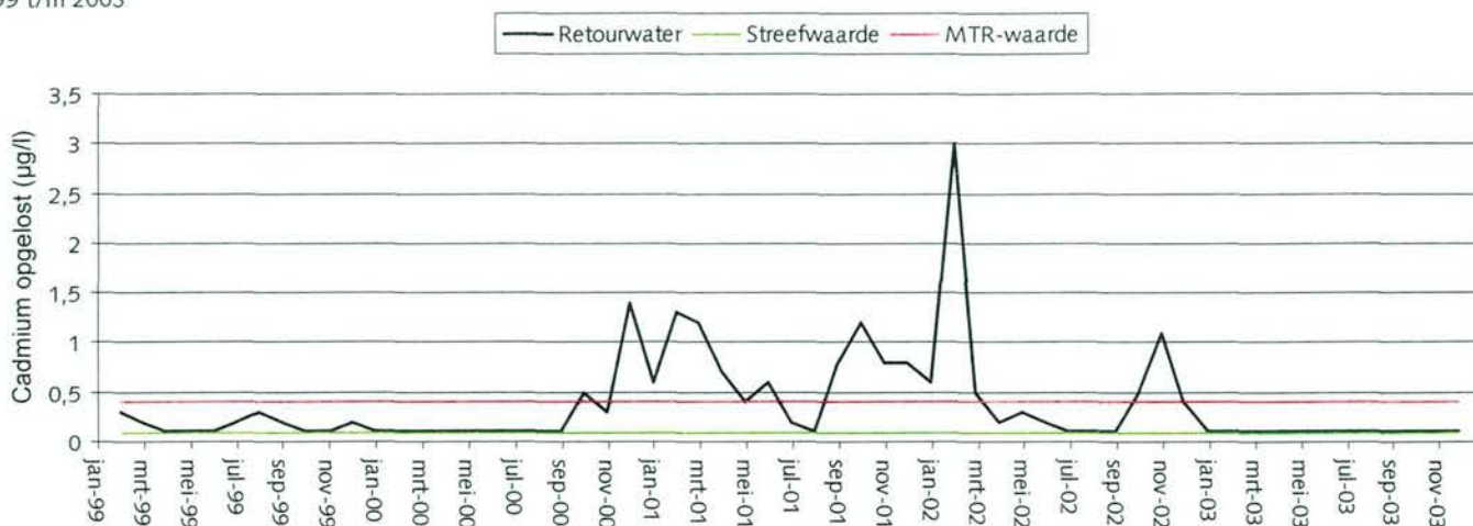
Figuur 16 Gidsparameter Cadmium (opgelost) 1999 t/m 2003
