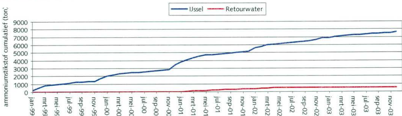
Figuur 10 Cumulatieve vrachten ammoniumstikstof van de IJssel en het retourwater vanaf 1999 t/m 2003
