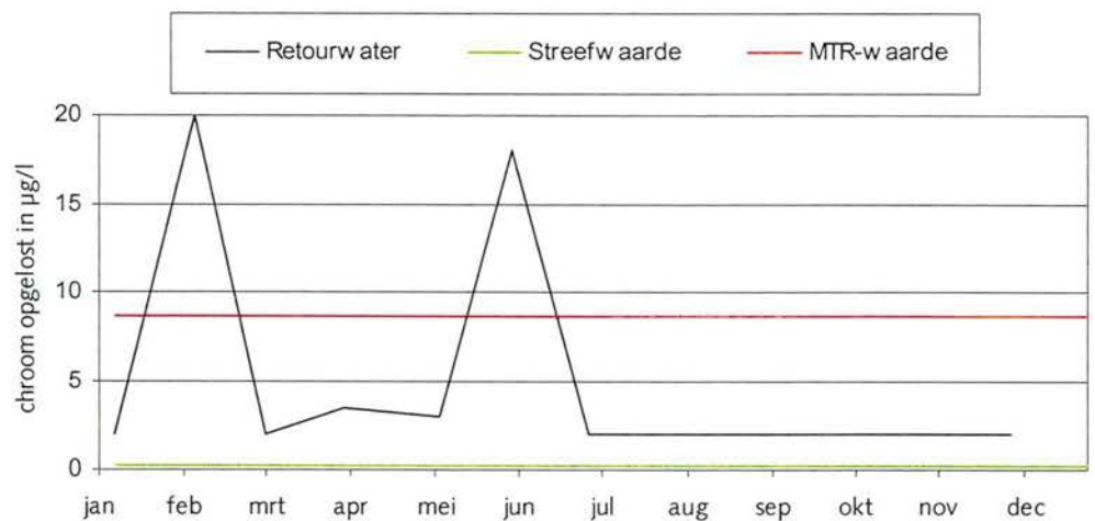
Figuur 18 Chroom opgelost in retourwater in 2003
