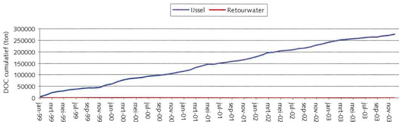
Figuur 15 Cumulatieve vrachten DOC van de IJssel het retourwater vanaf 1999 t/m 2003
