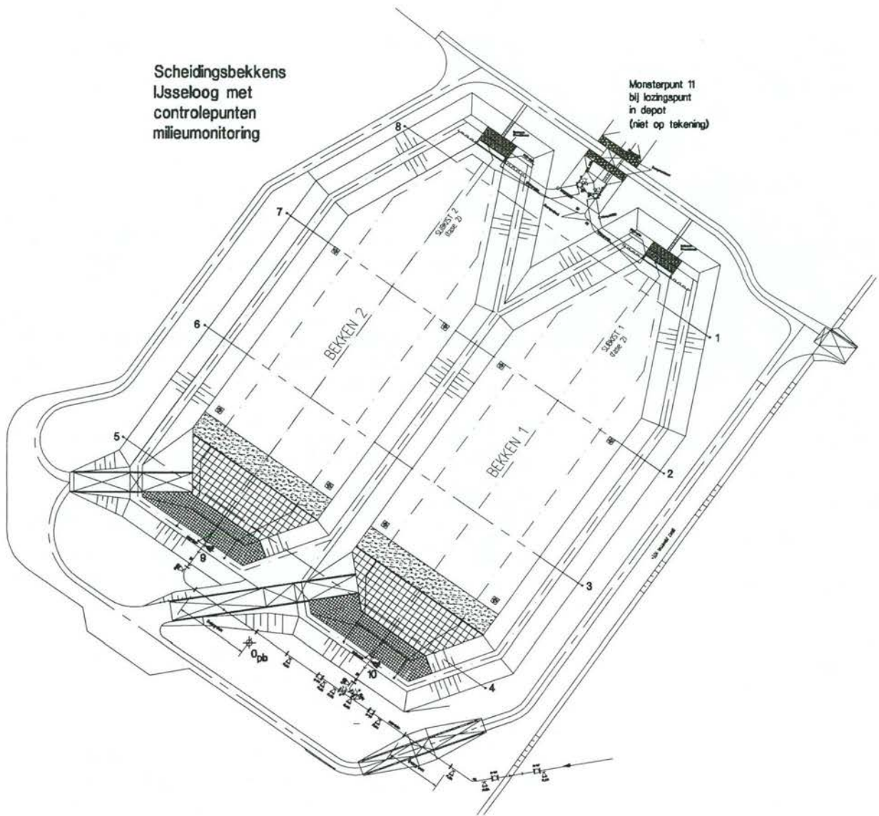
Figuur 23 Overzicht peilbuizen rondom scheidingsbekken 2
