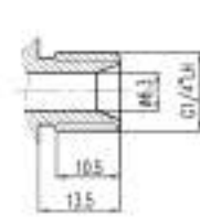
EN16129-H-4-G14/LH
