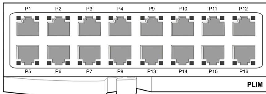
Рис. 2.19 Плата PLIM - вид спереди
