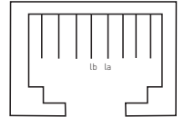
Belegung der UP0 Anschlüsse
