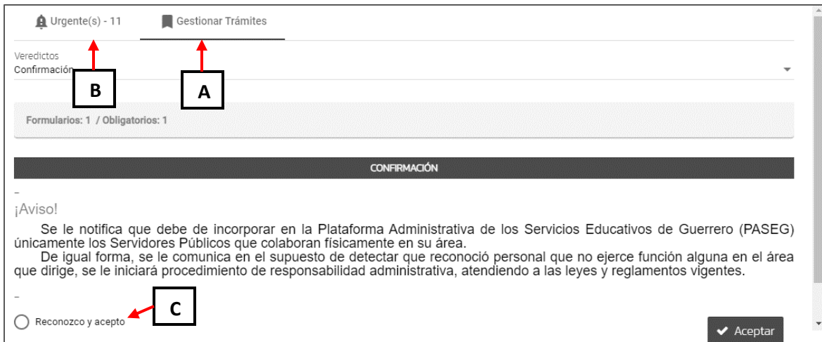
Imagen.1.4 Ventana emergente.
