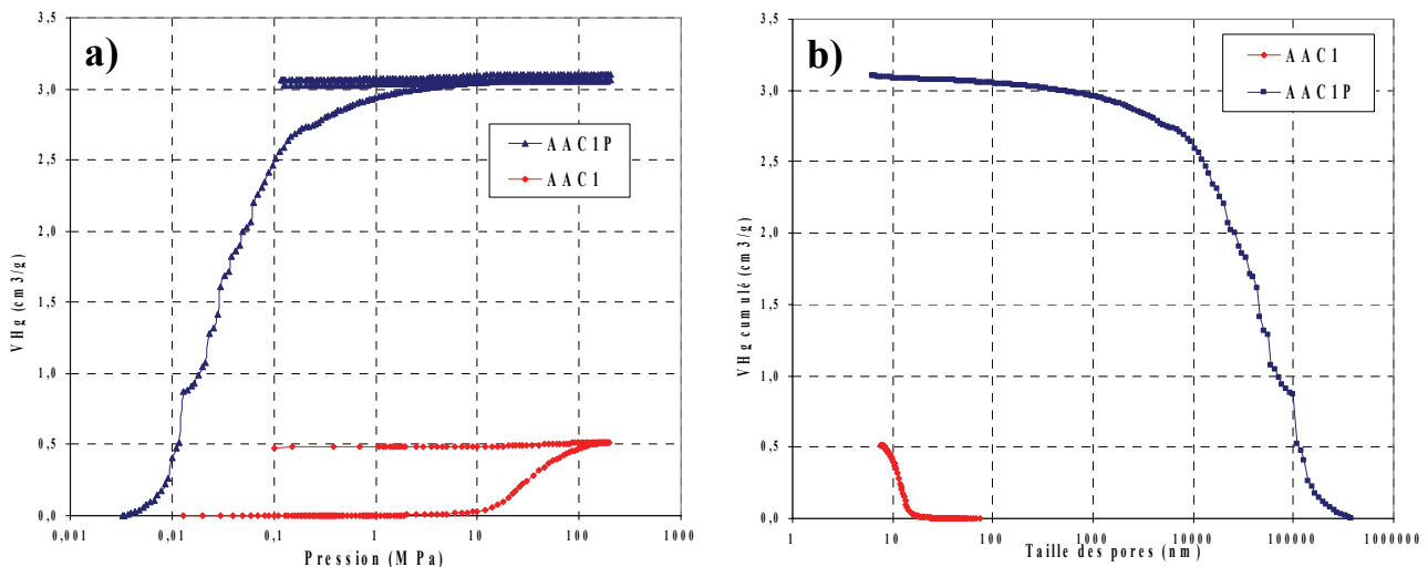
Figure IV-13: Comparaison de la porosité de AAC1 et AAC1P par porosimétrie mercure a) Volume poreux en fonction de la pression isostatique de mercure b) Volume poreux en fonction de la taille des pores
