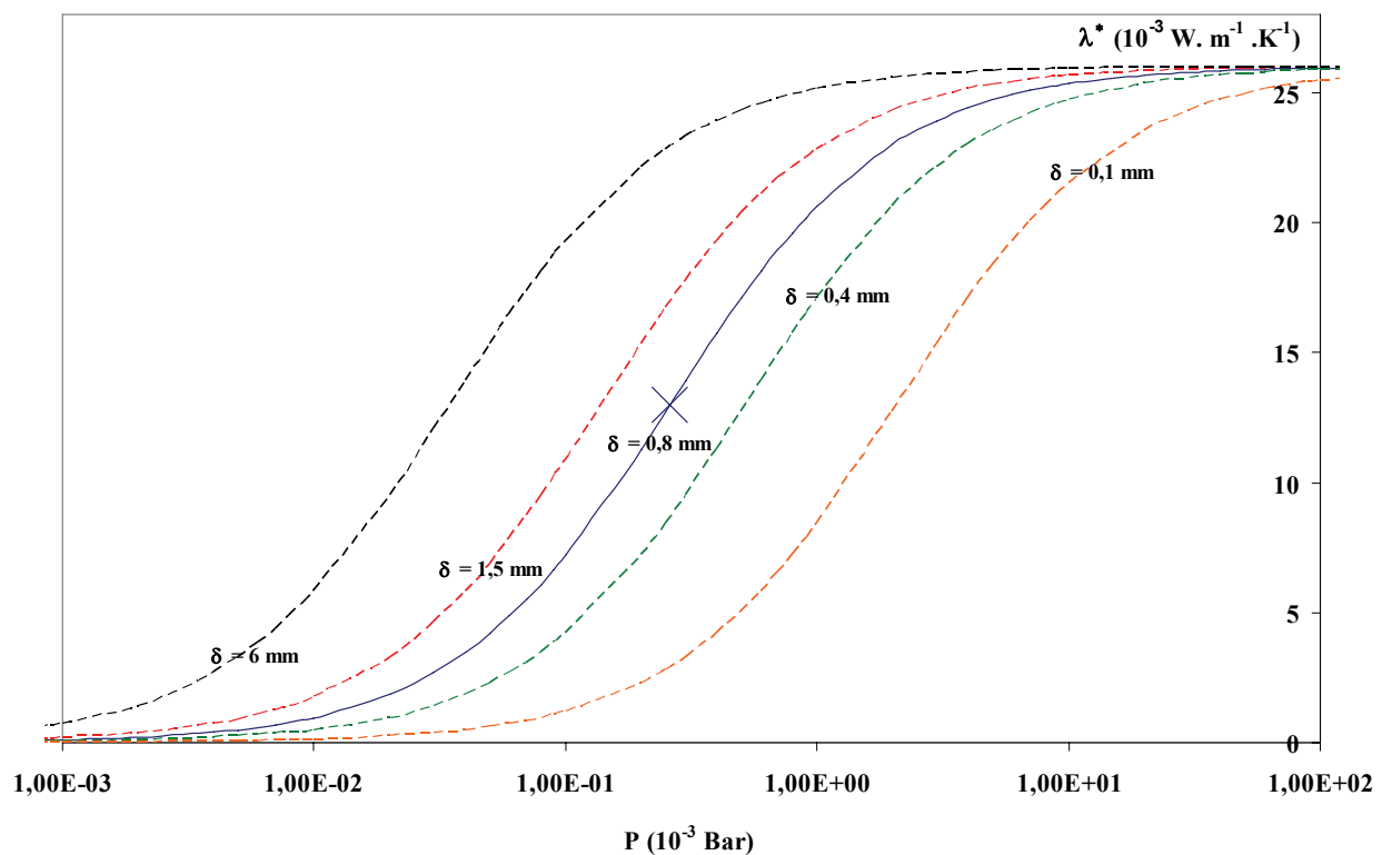
Figure A-12: Evolution de la conductivité thermique de l'air en fonction de la pression pour différentes dimensions de confinement
