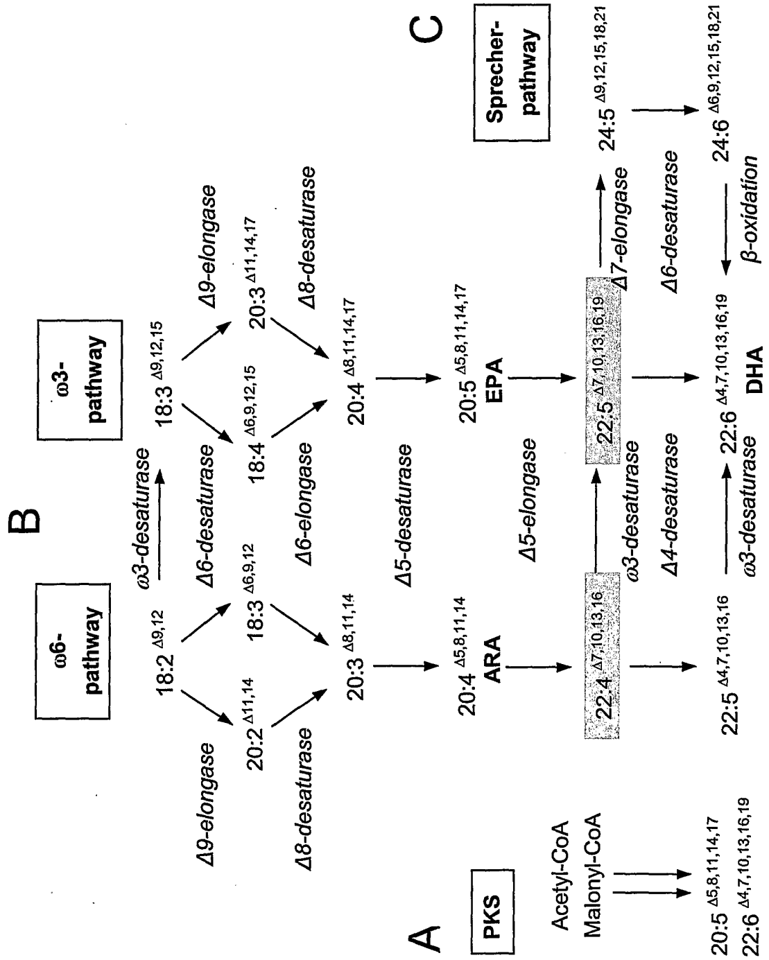
Figur 1: Verschiedene Synthese-Wege zur Biosynthese von DHA (Docosahexaensäure)
