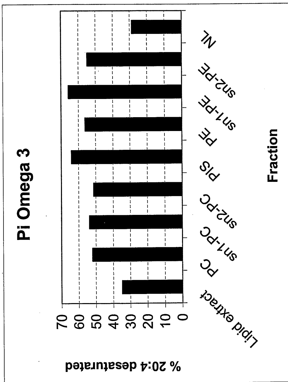
Figur 9: Desaturierung von Phospholipid gebundener Arachidonsäure zu EPA durch die Pi-Omega3Des
