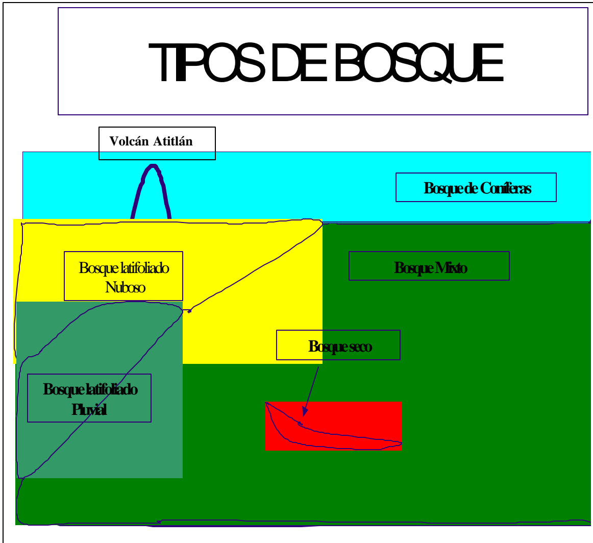
Figura 2: Distribución Altitudinal de los Diferentes Tipos de Bosque en el Área de Estudios
