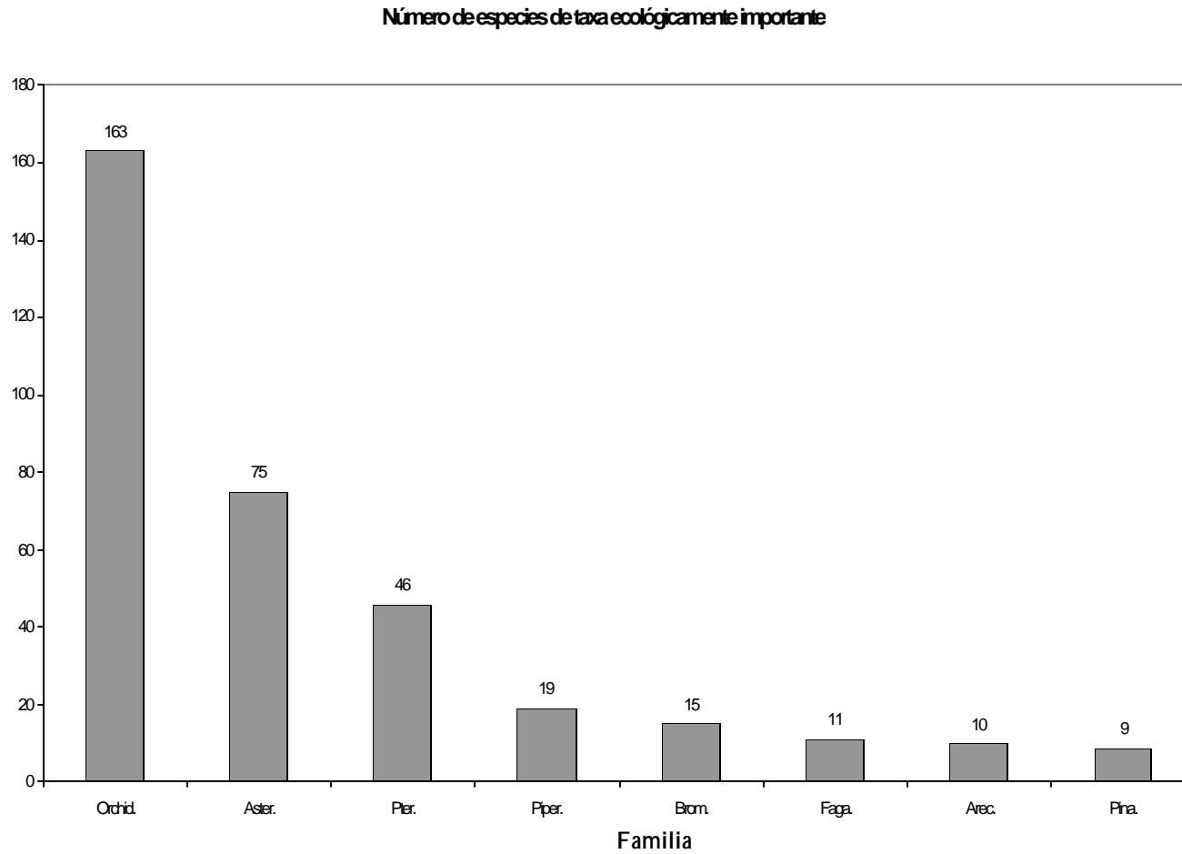
Figura 4: Estadísticas de la Flora de la Cuenca de Atitlán, Sololá
