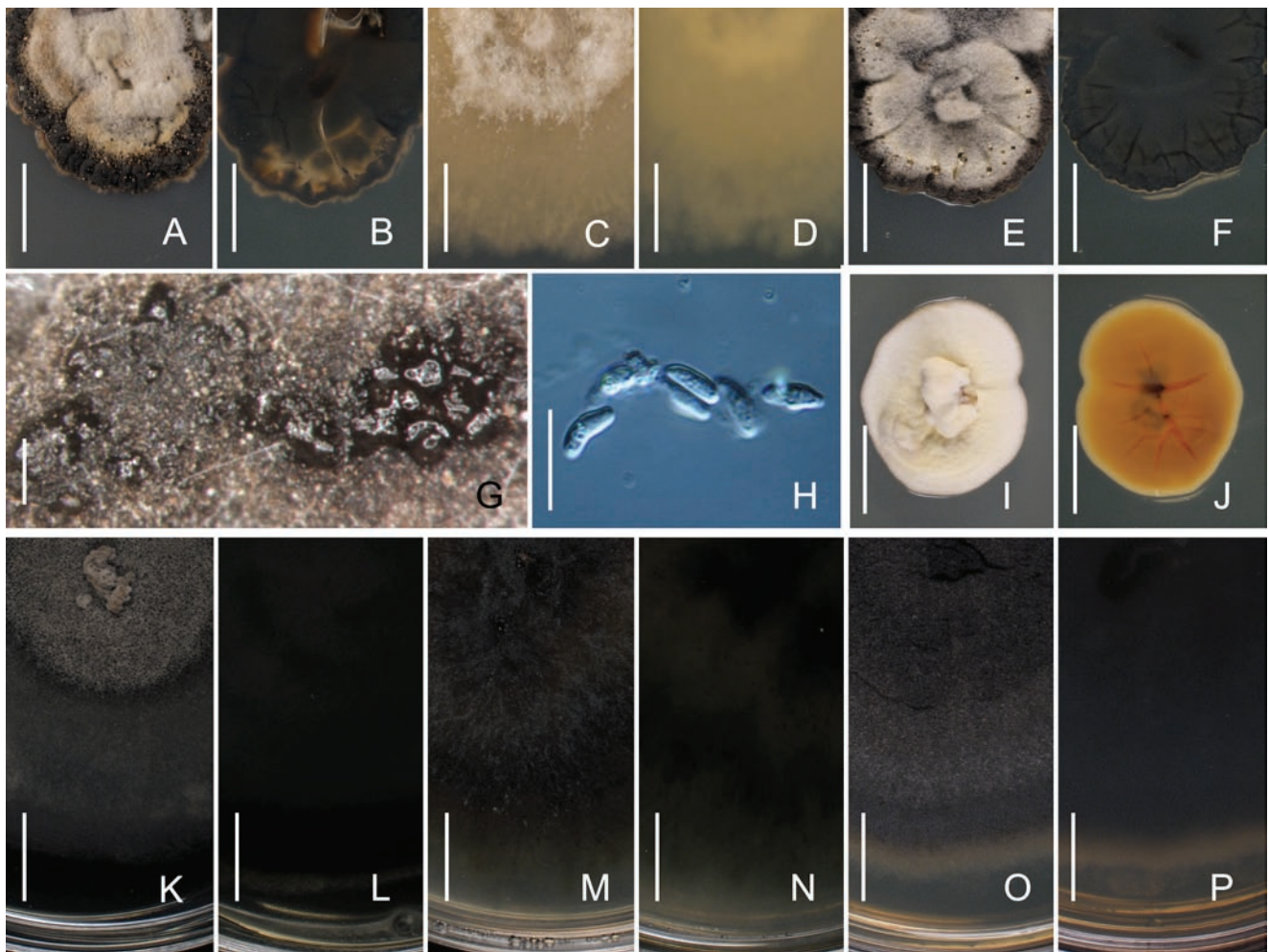
Fig. 8. Culture morphology. A–H. Gnomonia ostryae CBS 121242. I, J. G. pendulorum ex-type CBS 121264. K–P. G. rodmanii ex-type CBS 121909. A–F, I–P. Colony habit, 40 d, 23 °C. A, C, E, I, K, M, O. Surface. B, D, F, J, L, N, P. Reverse. G. Conidiomata, 4 mo, 2/10 °C. H. Conidia, 4.5 mo, 2/10 °C. A, B, G, H, K, L. PDA. C, D, M, N. MEA. E, F, I, J, O, P. MYA. Scale: A–F, I–P. 1 cm. G. 200 µm. H. 10 µm.
