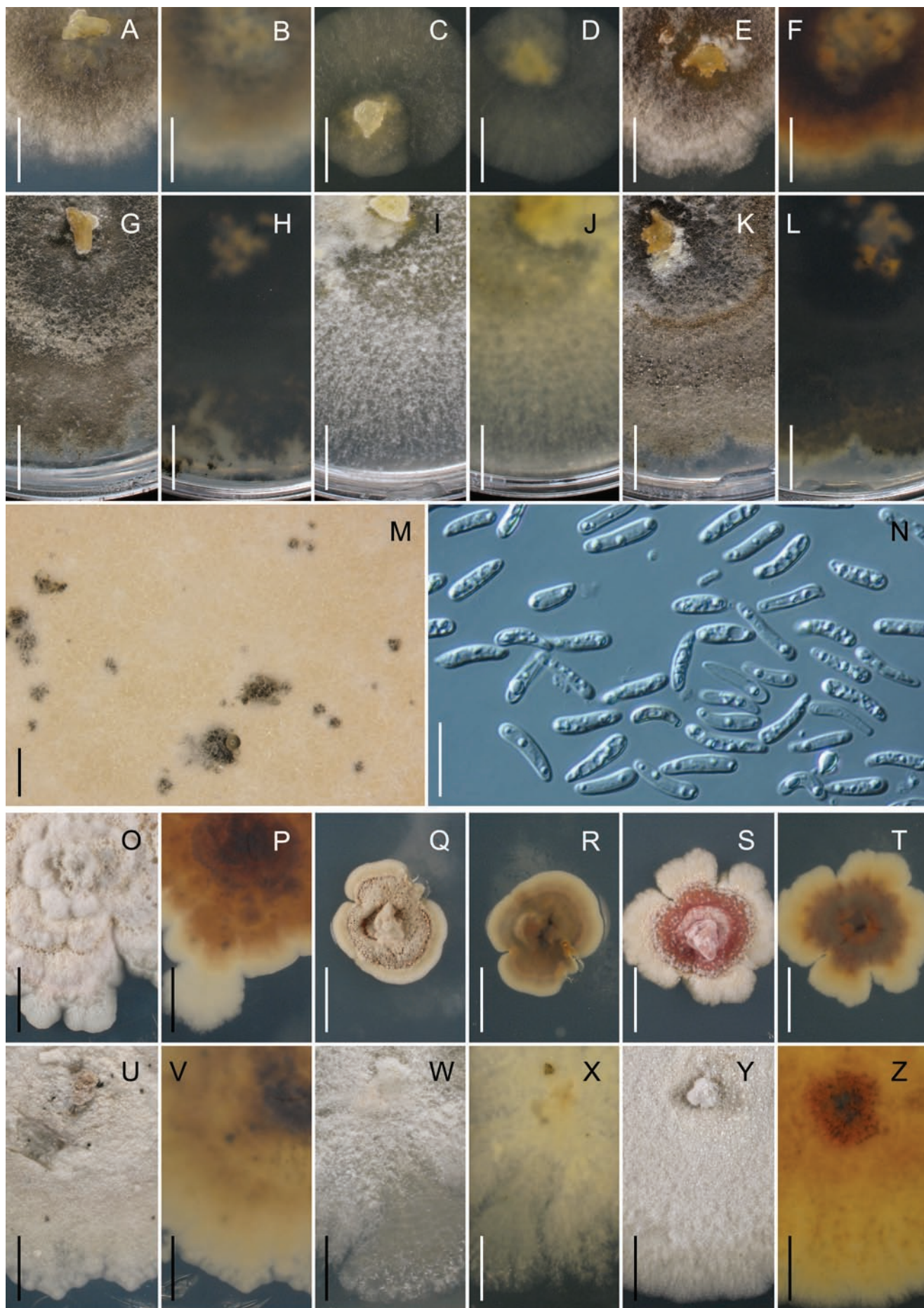
Fig. 30. Culture morphology. A–N. Ophiognomonia balsamiferae ex-type CBS 121266. O–Z. O. pseudoclavulata . O–T. Ex-type CBS 121236. U–Z. CBS 121232. A–L, O–Z. Colony habit. A, C, E, G, I, K, O, Q, S, U, W, Y. Surface. B, D, F, H, J, L, P, R, T, V, X, Z. Reverse. M. Conidiomata. N. Conidia. A–F. 14 d, 23 °C. G–Z. 40 d, 23 °C. A, B, G, H, O, P, U, V. PDA. C, D, I, J, M, N, Q, R, W, X. MEA. E, F, K, L, S, T, Y, Z. MYA. Scale: A–L, O–Z. 1 cm. M. 200 µm. N. 10 µm.
