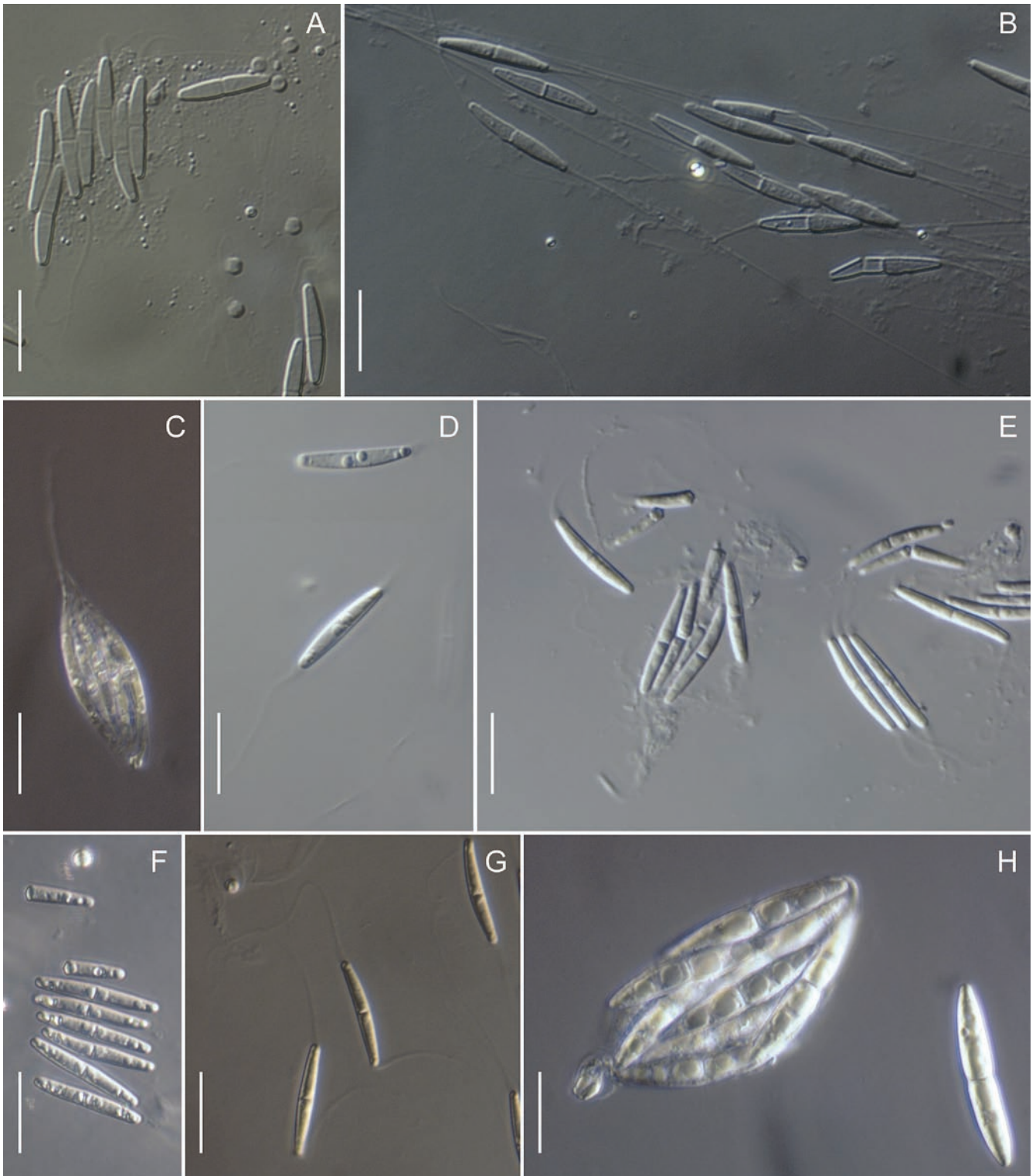
Fig. 36. Morphology on natural substrates, asci and ascospores. A, B. Ophiognomonium ischnostyla . A. BPI 877514B. B. BPI 877619. C–H. O. cf. ischnostyla . C, D. BPI 877605A. E. BPI 877605B. F. BPI 877467B. G. BPI 877622. H. BPI 877616. Scale 10 \mu m.
