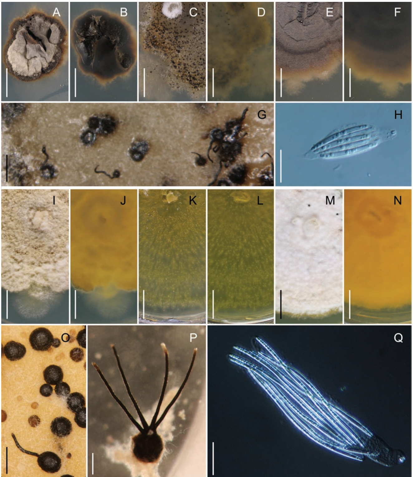
Fig. 39. Culture morphology. A–H. Ophiognomonia rosae CBS 121263. I–Q. O. sassafras CBS 121243. A–F, I–N. Colony habit, 40 d, 23 °C. A, C, E, I, K, M. Surface. B, D, F, J, L, N. Reverse. G, O, P. Perithecia. H, Q. Asci. G, H. 40 d, 23 °C. O–Q. 4.5 mo, 2/10 °C. A, B, I, J, P. PDA. C, D, G, H, K, L, Q. MEA. E, F, M, O. MYA. Scale: A–F, I–N. 1 cm. G, O. 500 µm. P. 200 µm. H, Q. 10 µm.
