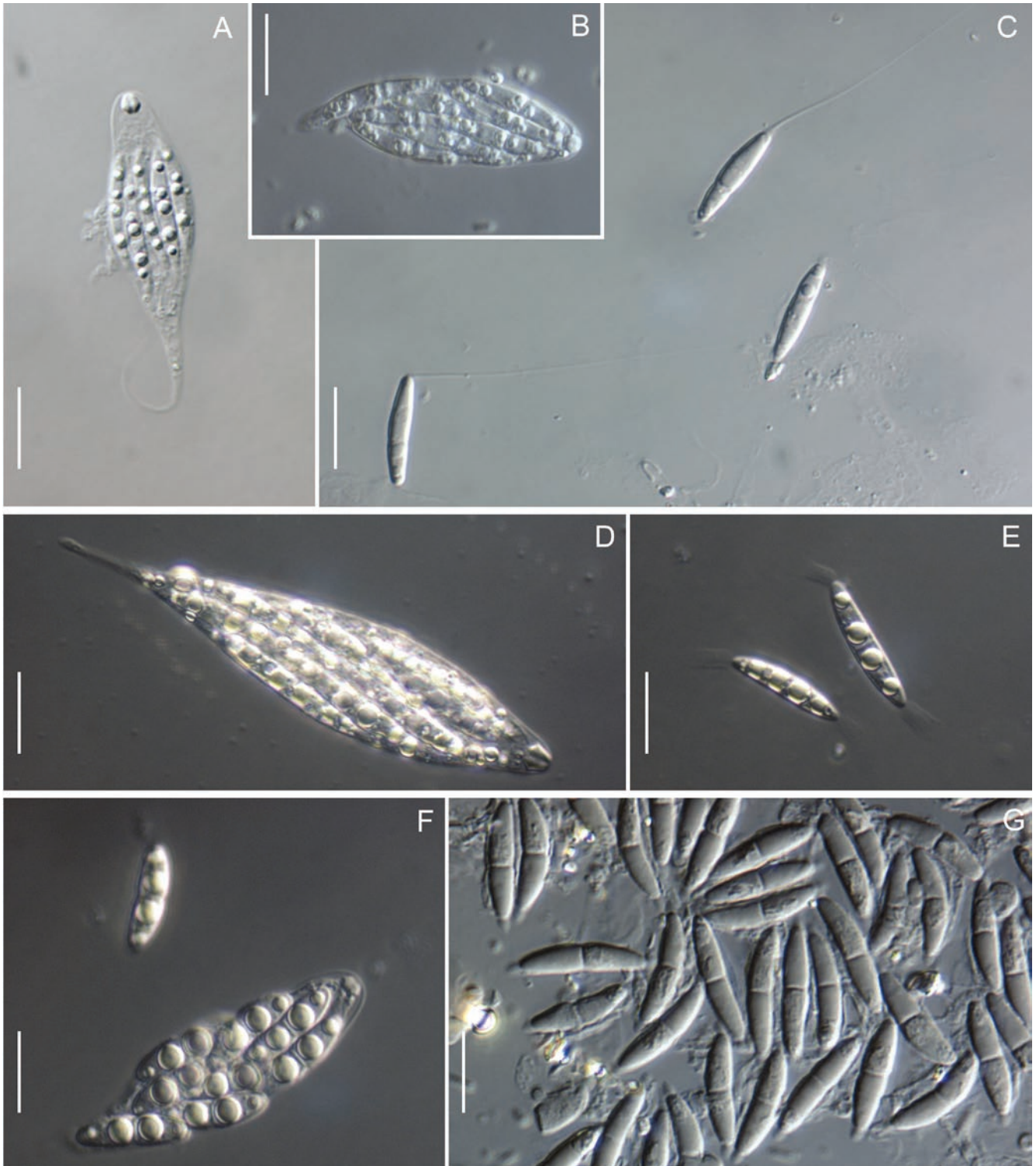
Fig. 13. Morphology on natural substrate, asci and ascospores. A–C. Gnomonia virginianae . A. BPI 877565A. B. Holotype BPI 844264. C. BPI 878209. D, E. G. amoena , BPI 877469. F, G. G. pseudoamoena . F. BPI 877518. G. Stirpes Cryptogamae Vogeso-Rhenanae 1251, BPI bound. Scale 10 \mu m.
