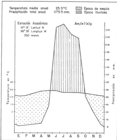
Fig. 2. Diagrama ombrotérmico de Acazónica, Ver.
