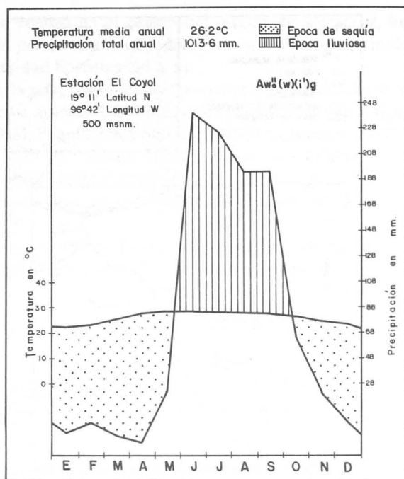
Fig. 3. Diagrama ombrotérmico de El Coyal, Ver.
