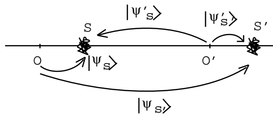
FIG. 3.1 - Premier point de vue actif dans le cas d'une translation. Les conventions sont telles que, par exemple, on appelle |\psi_S\rangle le ket attribué par \mathcal{O} au système S et |\psi'_{S'}\rangle = U|\psi_S\rangle celui attribué par \mathcal{O}' au même système, U faisant le passage entre \mathcal{O} et \mathcal{O}'
