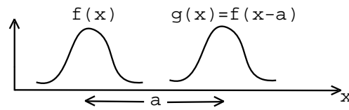
FIG. 3.2 - Dans une translation de +a , la fonction traduite g(x) vaut f(x-a)
