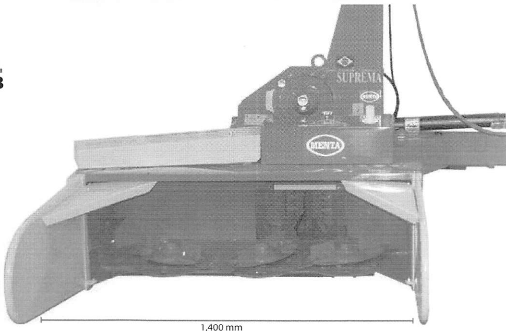
PMCD 1.3 - Plataforma recolhadora de capim e gramíneas plantados em área total, com 3 discos de corte. Plataforma cosechadora de pasto y gramíneas en área total, con 3 (tres) discos de corte.
