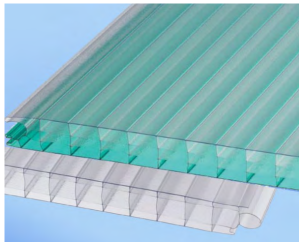
Doppelsteg-Wand-Elemente zum stecken
