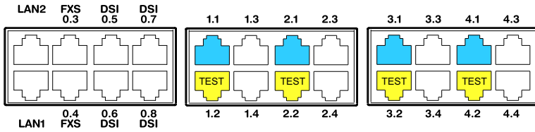
Fig. 35 Anschlussmöglichkeiten PRI-Netzschnittstellen
