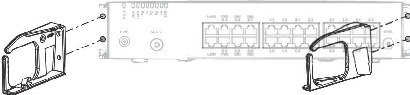
Fig. 18 Montage der Halter für die Kabelabdeckung
