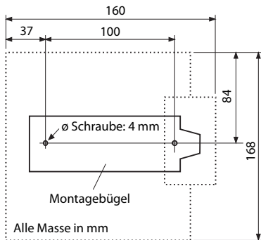
Fig. 65 Massbild für Wandmontage des Montagebügels
