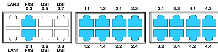
Fig. 52 Anschlussmöglichkeiten FXS-Endgeräteschnittstellen
