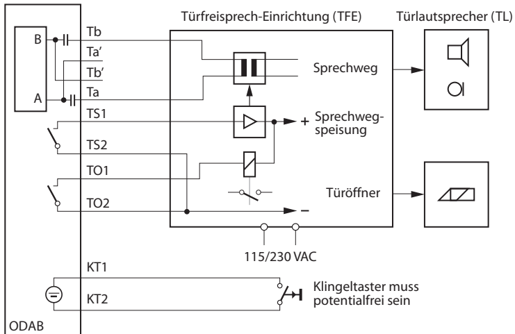
Fig. 60 Prinzip-Schema
