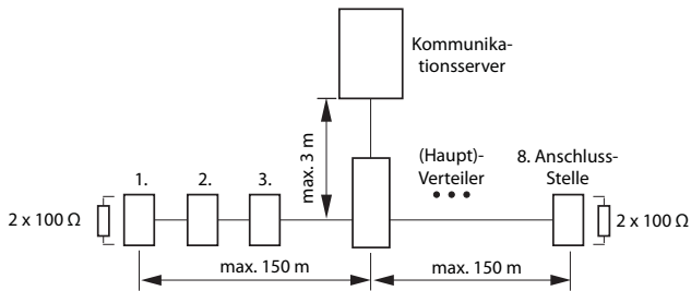
Fig. 47 S-Bus kurz, V-förmig
