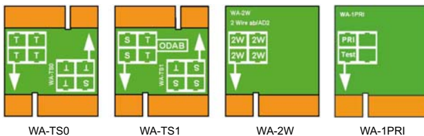
Fig. 10 Verdrahtungsadapter-Typen
