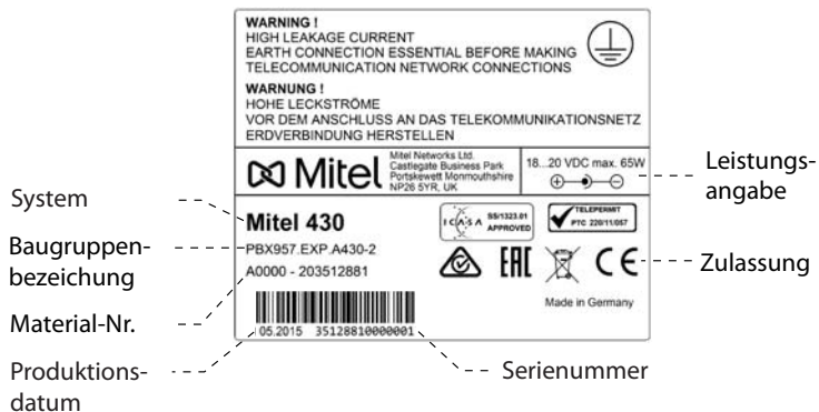
Fig. 80 Typenschild (Beispiel Kommunikationsserver Mitel 430)
