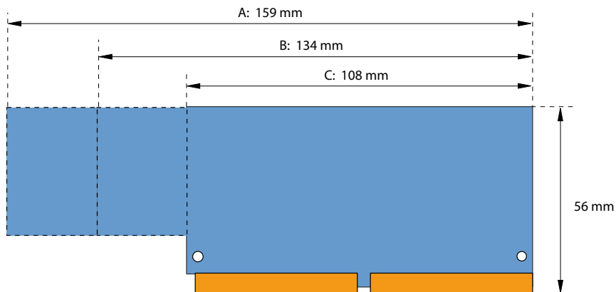
Fig. 82 Abmessungen Schnittstellenkarten (Bauform A, B, C)
