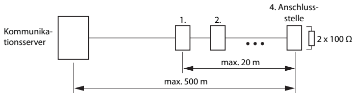
Fig. 48 S-Bus, lang
