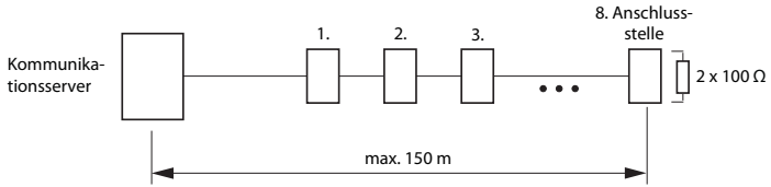
Fig. 46 S-Bus kurz
