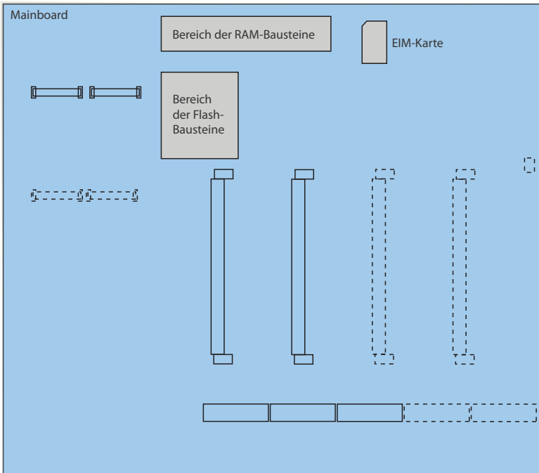
Fig. 73 Speicher auf dem Mainboard Mitel 415/430
