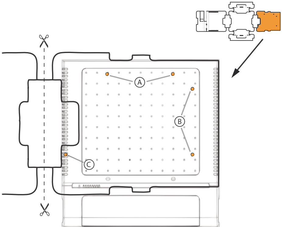
Fig. 15 Bohrschablone
