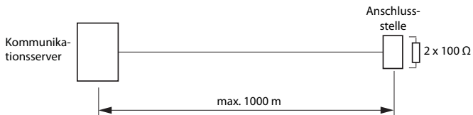
Fig. 49 S-Bus, Punkt-Punkt
