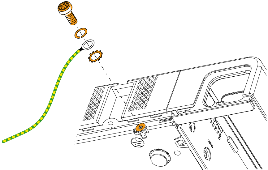
Fig. 19 Erdungsanschluss
