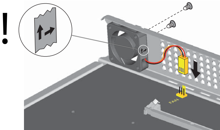
Fig. 17 Einbau des Lüfters in Mittel 430
