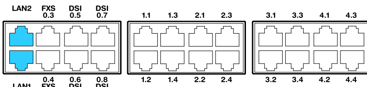
Fig. 63 Anschlussmöglichkeiten Ethernet-Schnittstellen
