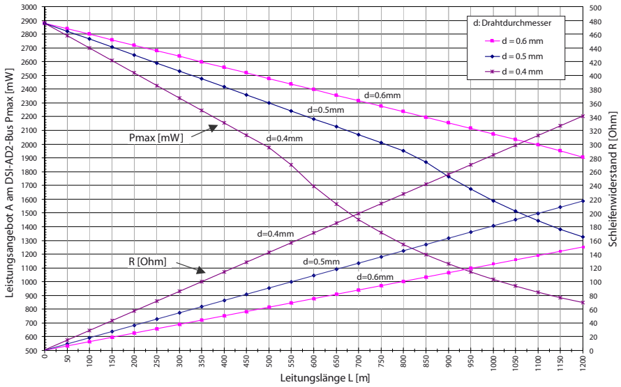
Fig. 43 Verfügbare Leistung Fall A am DSI-AD2-Bus
