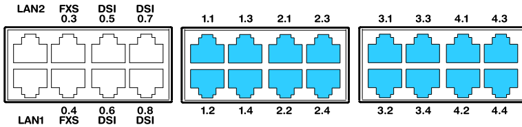
Fig. 31 Anschlussmöglichkeiten BRI-Netzchnittstellen
