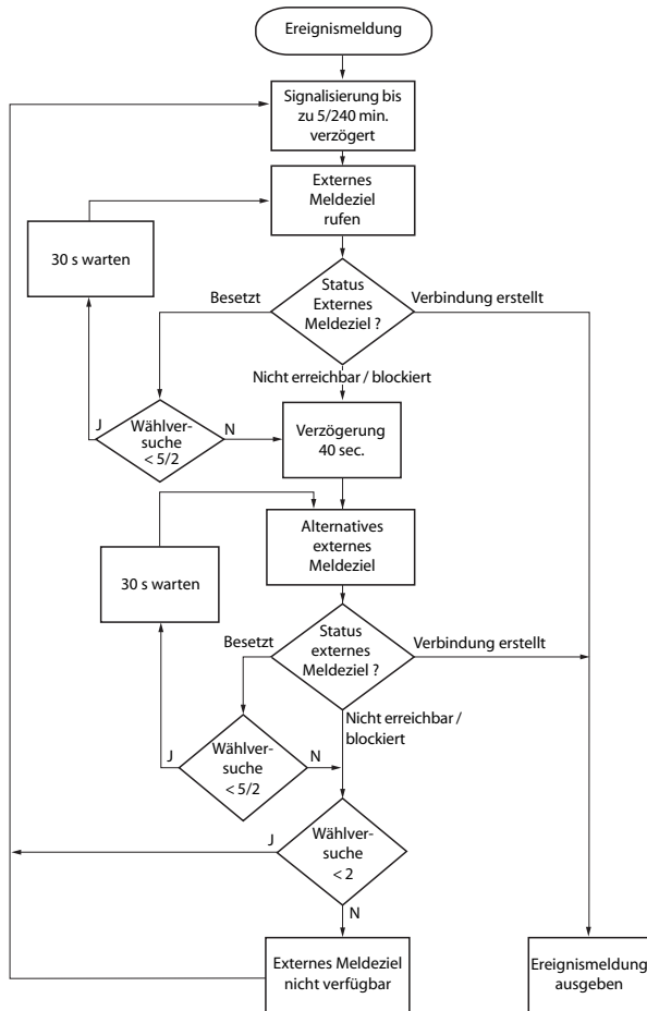
Fig. 79 Flussdiagramm Signalisierung einer Ereignismeldung an ein externes Meldeziel
