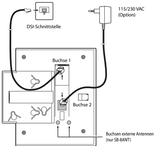
Fig. 67 Rückseite der Funkeinheiten mit Anschluss-Stellen
