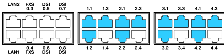
Fig. 45 Anschlussmöglichkeiten BRI-S-Endgeräteschnittstellen
