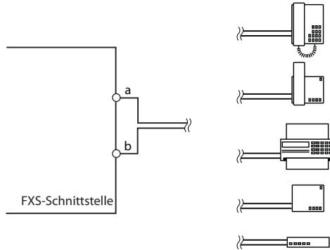
Fig. 53 Beschriftung für FXS-Modus: Telefon/Fax
