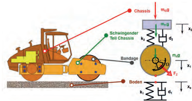
Abbildung 2. Analytisches Modell eines Verdichtungsgerätes mit unwuchterregter Bandage und schwingendem Chassisanteil (ein Teil schwingend, ein Teil statisch/stationär)
