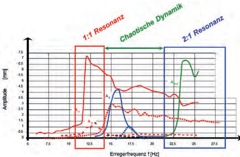
Abbildung 4. Gemessene Schwingungen eines Walzenzugs mit teilweise mitschwingendem Chassis, welches als Tilger wirkt. Die Messungen wurden auf sandig-kiesigem Boden in Spanien durchgeführt. A_i bezeichnet die Amplitude des Schwingungsanteils mit der Frequenz i \cdot f , wobei f die Erregerfrequenz bedeutet.
