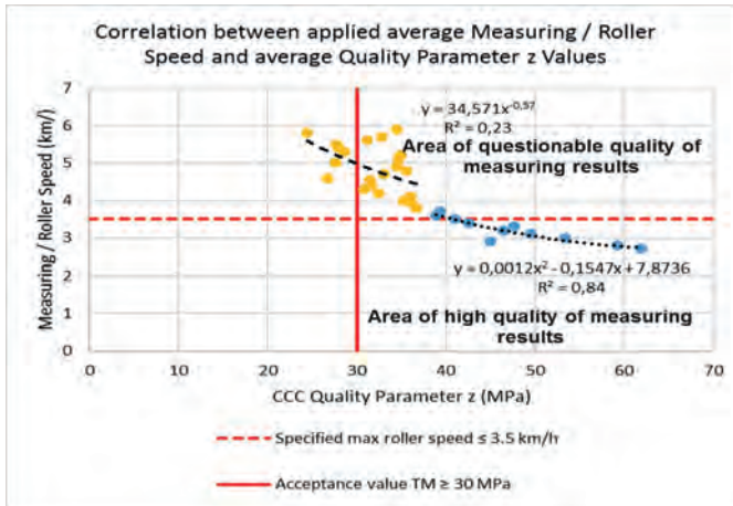
Abbildung 5. Zusammenhang zwischen Walzen- bzw. Verdichtungsgeschwindigkeit und Verdichtungserfolg.
