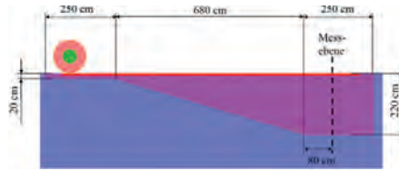
Abbildung 5. Aufbau einer Verdichtungsbahn mit ansteigender Schichtdicke
