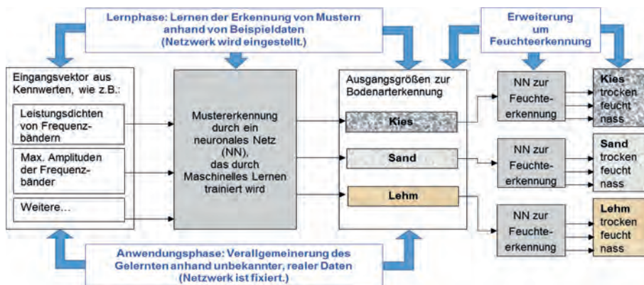
Abbildung 3. Ablauf des maschinellen Lernens am Beispiel hintereinandergeschalteter Neuronaler Netze
