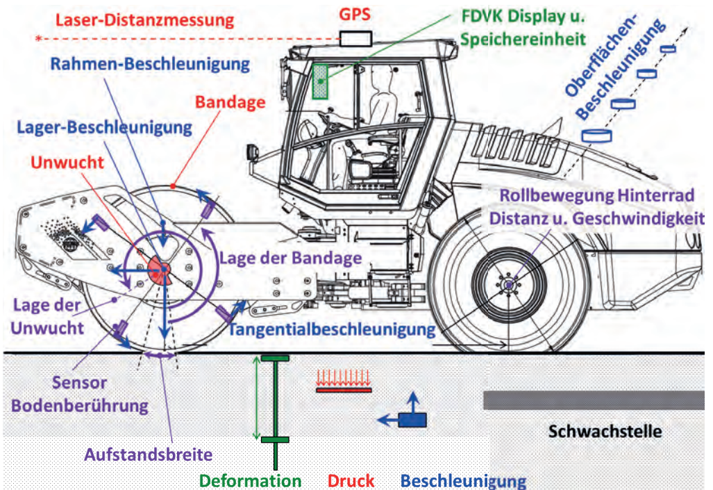
Abbildung 1. Mögliche messtechnische Instrumentierung des Walze-Boden-Interaktionssystems.
