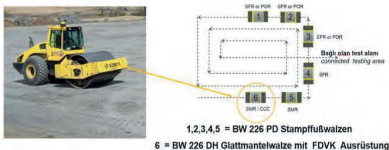
Abbildung 4. Walzschema für 6 im Kreis fahrende Walzenzüge.
