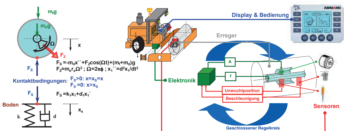
Abbildung 1. Modell einer klassischen Vibrationswalze samt zugehörigem Mess- und Regelsystem.
