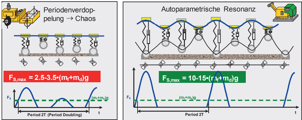
Abbildung 3. Tilgereffekt einer schwingenden Chassismasse, eine Leistungssteigerung von rund 400% ist realisierbar. Gut erkennbar die statische Wirkung des Chassis heutiger Maschinen und die Dynamik bei der Ausnutzung der autoparametrischen Resonanz
