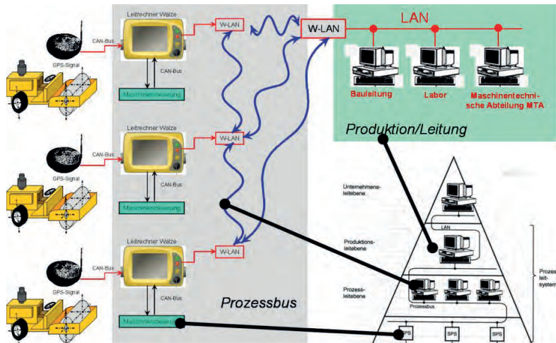
Abbildung 7. Zukunft der Verdichtungs-technologie – Maschinen werden vernetzt, ein modernes Bauunternehmen wird zu einer digitalen Fabrik – Strassenbau 4.0
