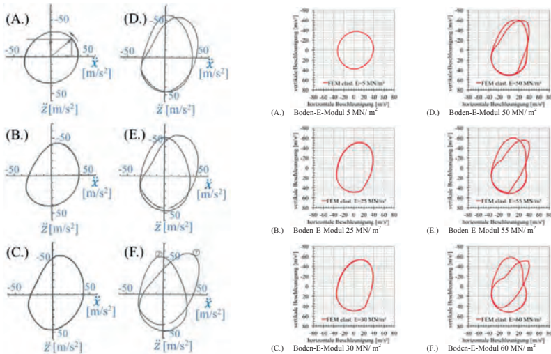
Abbildung 2. Bandagenbeschleunigungen – Vergleich von Messergebnissen (Kröber, 1988) (links) mit Berechnungsergebnissen (rechts).
