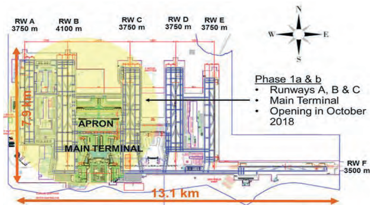
Abbildung 1. Neuer dritter Flughafen von Istanbul.
