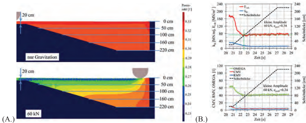
Abbildung 6. (A.) Porenzahlverläufe und (B.) Verläufe der verschiedenen FDVK-Werte über der Schichtdicke bei der Überfahrt mit der Vibrationsbandage einer HAMM HD+90 VO mit kleiner Amplitude.
