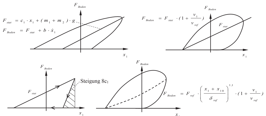
Abbildung 1. Kennlinien für Modelle A (oben links), B (oben rechts), C (unten links), D (unten rechts)
