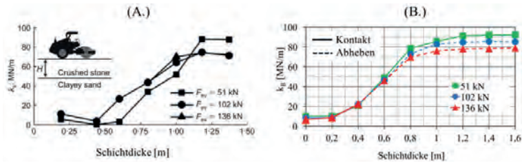
Abbildung 3. Verläufe des k_B -Wertes in Abhängigkeit von der Schichtdicke und der Erregerkraft – Vergleich von (A.) Messergebnissen (Rinehart 2008) und (B.) Berechnungsergebnissen.
