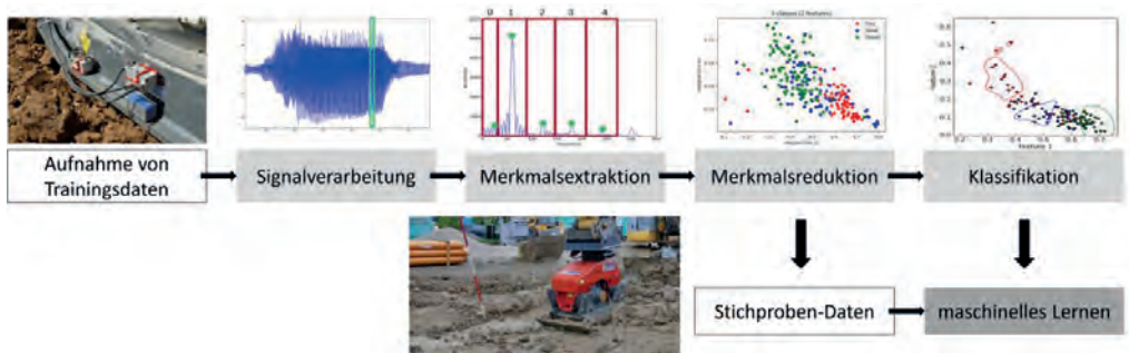
Abbildung 2. Schematischer Ablauf des maschinellen Lernens
