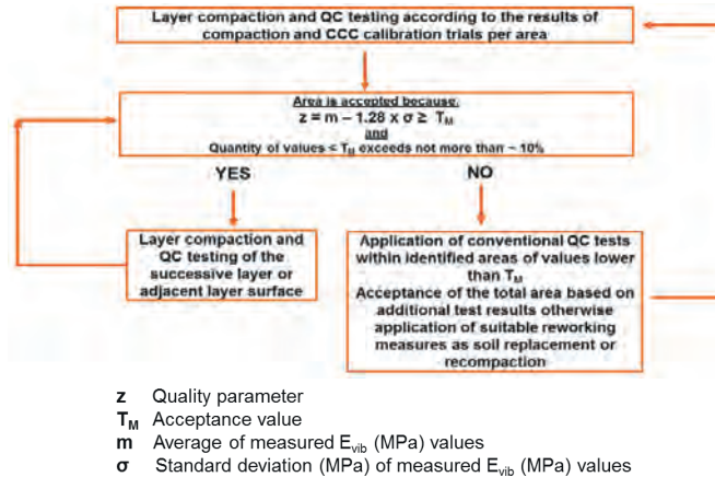
Abbildung 3. Arbeitsablauf zur Überwachung der Qualität verdichteter Lagen bei Einsatz der FDVK als Hauptprüfmethode.
