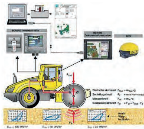
Abbildung 1. Messprinzip und Ausrüstung einer FDVK Walze.
