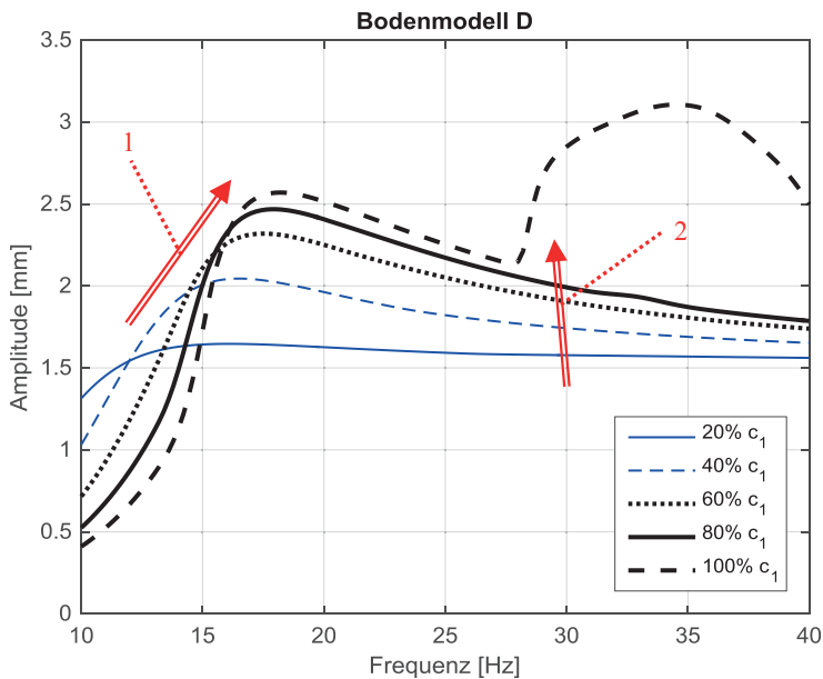
Abbildung 2. Amplitude über Frequenz, Parameter c_1
