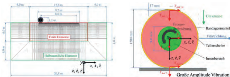
Abbildung 1. Allgemeiner Aufbau des Berechnungsmodells.
