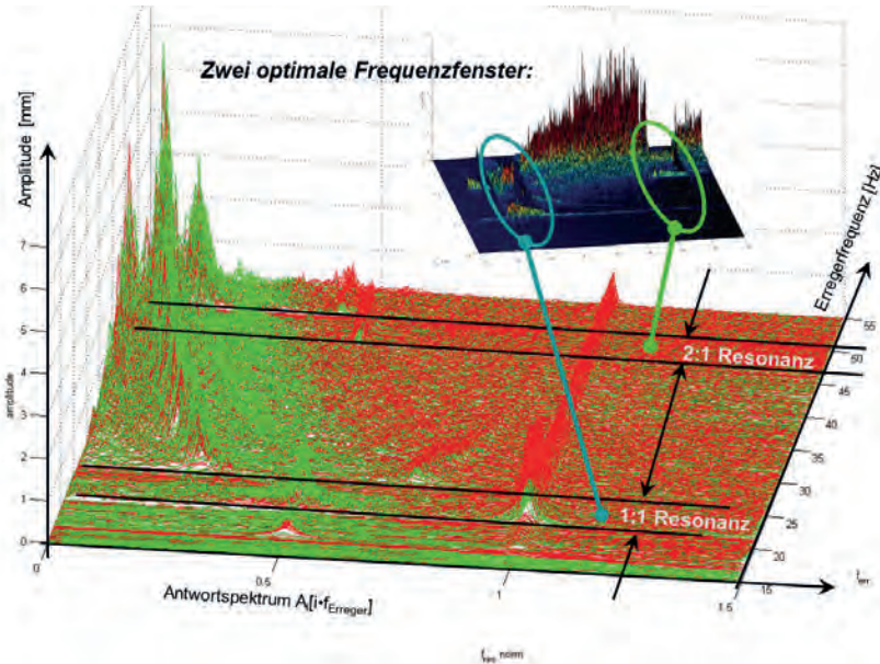
Abbildung5. Übersicht über das Frequenzspektrum eines Walzenzugs in Abhängigkeit der Erregerfrequenz der Maschine. Gut zu erkennen ist das Schwingungssignal mit der Anregungsfrequenz f_{\text{Erreger}} , sowie die 1:1- und die 2:1-Resonanzzone. Diese beiden Frequenzbereiche sind stabil, alle andern entsprechen chaotischem Verhalten.
