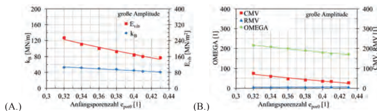
Abbildung 4. Verläufe der verschiedenen FDVK-Messwerte in Abhängigkeit von der Anfangsporenzahl.
