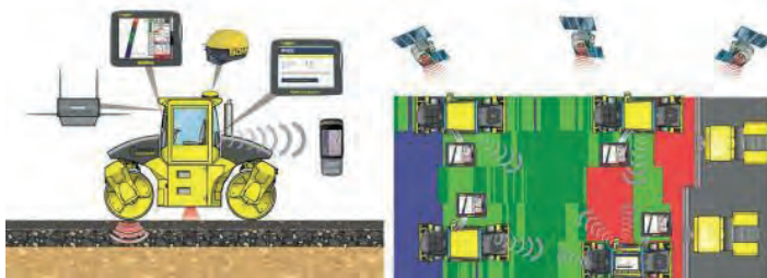
Abbildung 3. Vernetzung von mehreren Walzen zur Prozessdokumentation im Asphaltbau.
