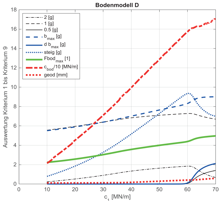
Abbildung 3. Abhängigkeit aller Kriterien für Bodenmodell D.
