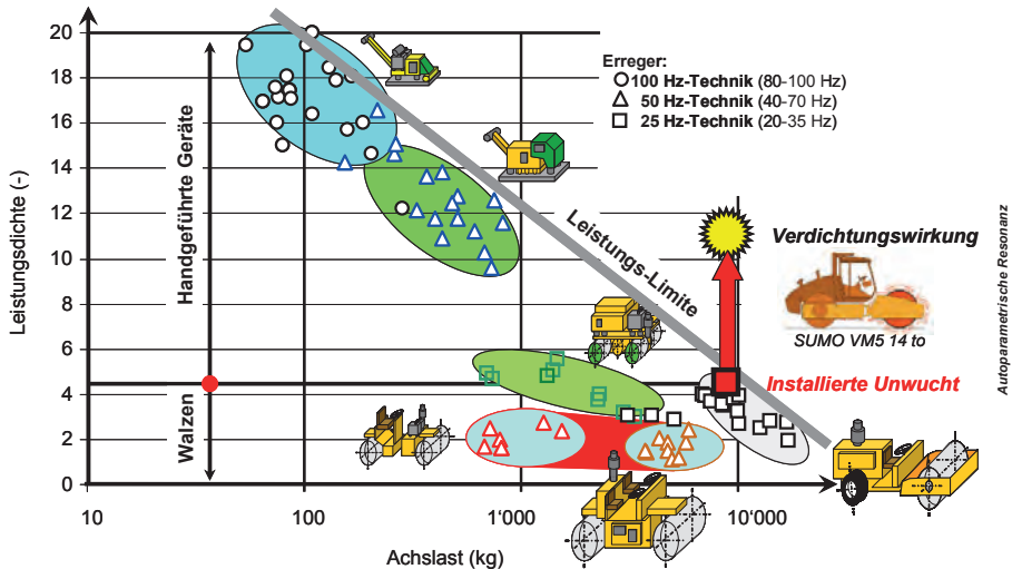
Abbildung 6. Klassifikation der Verdichtungsgeräte, dargestellt in halblogarithmischem Massstab. Die “Leistungs-dichte” bezeichnet den Quotienten von Zentrifugalkraft und schwingender Masse (in kN).
