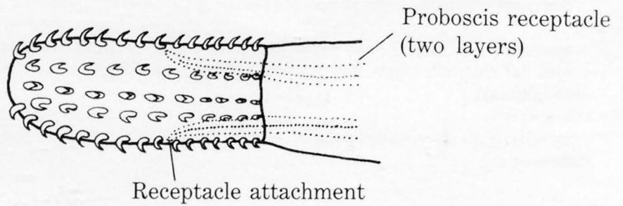
1.3 Centrorhynchus
