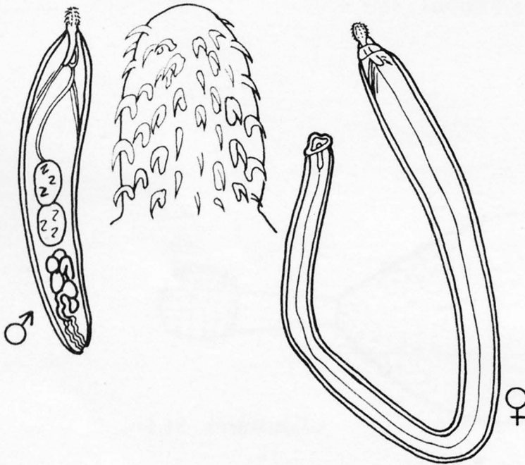
2.3 A. ranae
