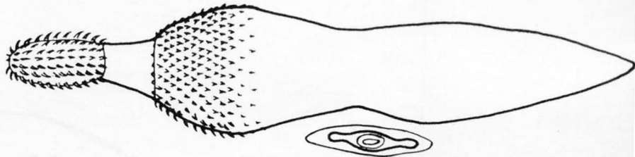
1.9 Polymorphus
