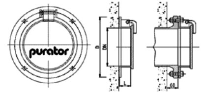
Wandbefestigung mit Dübel Flanschverbindung (Flanschtyp: PN10)
