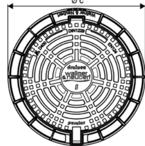
Variante hochziehbarer Rahmen
