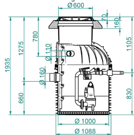
Belastungsklasse B125
