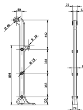
Ausführung OW14
