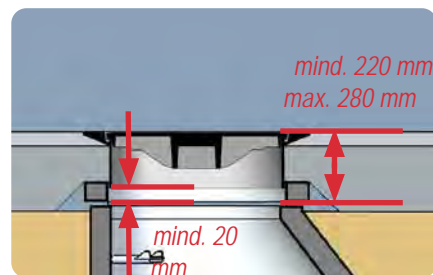
Einbau DRAINEX Niveau mit Adapting
