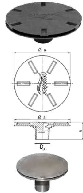
Variante Komplett-Edelstahl auf Anfrage
