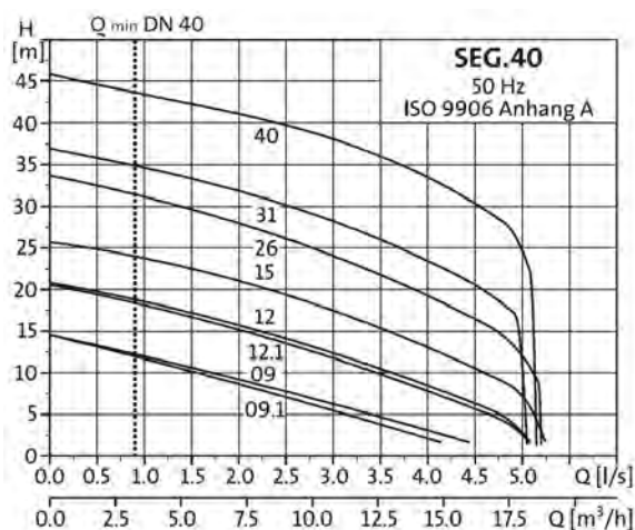
Typen SEG.40
