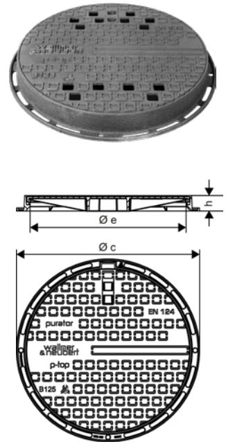
Variante Beton-Gussrahmen
