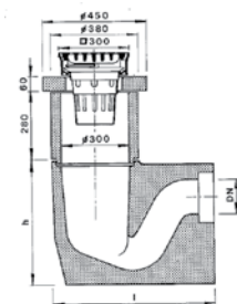
mit Geruchsverschluss
