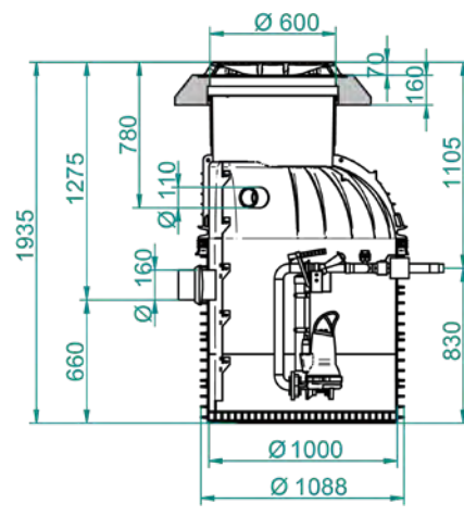
Belastungsklasse B125
