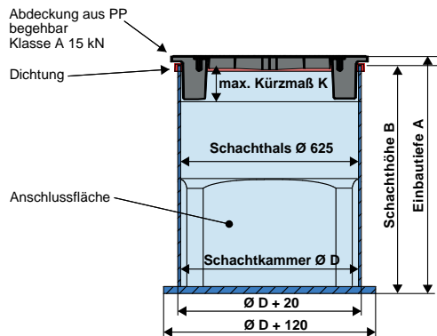
Einbauschema mit Kunststoffabdeckung Klasse A 15 begehbar
