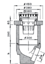
ohne Geruchsverschluss
