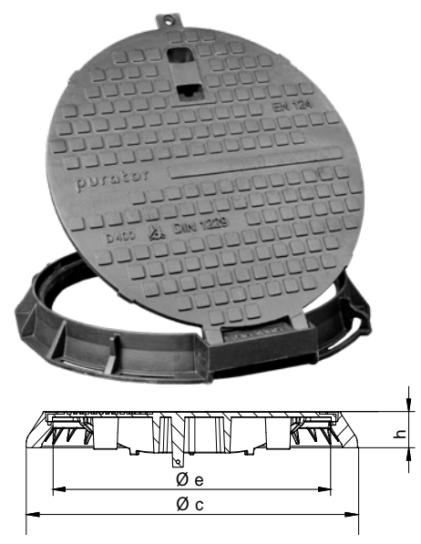
P-TOP® Strong 800 mit Gasdruckfeder
