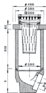
ohne Geruchsverschluss
