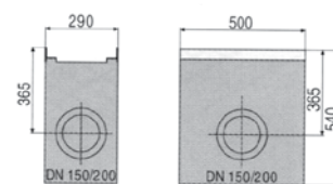
Einlaufkasten
