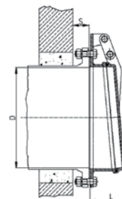
Flanschverbindung (Flanschtyp: PN10)
