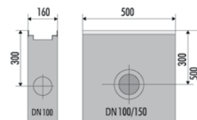
Einlaufkasten FFX8053
