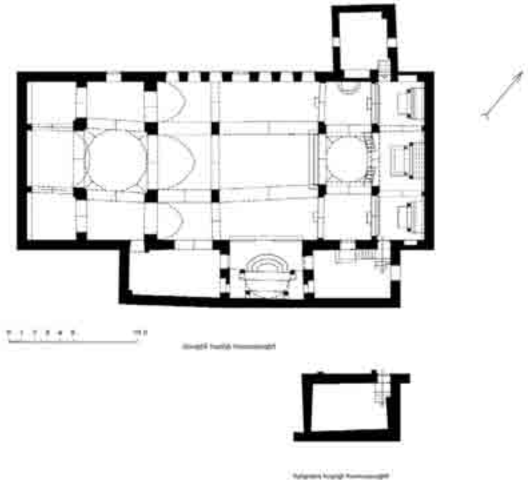
Եկեղեցու հատակագիծը երկու հարկերով (չափ.՝ 01.12.2010)
