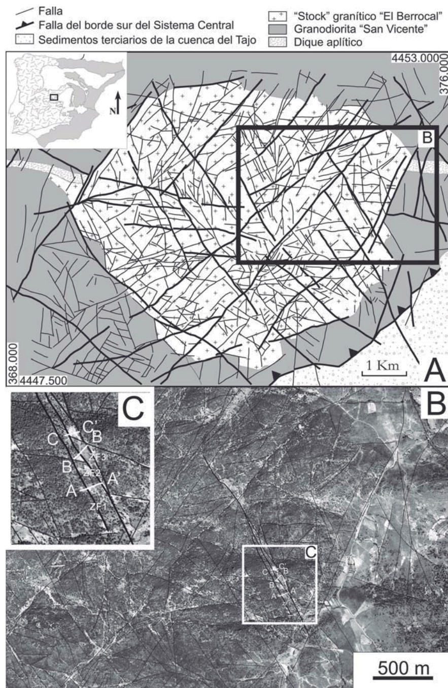
Fig. 1.- A) Localización y mapa geológico de la zona de estudio. B) Mapa de fracturación del borde Oriental del macizo de El Berrocal sobre la ortoimagen 1:2000. C) Detalle de la fracturación y localización de las tres secciones de tomografía realizadas.
