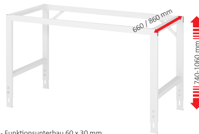
Grundtischgestell Tom- Funktionsunterbau 60 x 30 mm Höhenverstellung von 740-1060 mm
