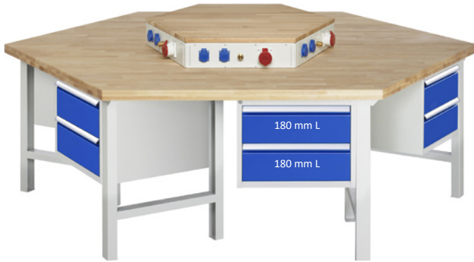
Buche-Massiv-Arbeitsplatte mit Kantenlänge 1350 mm (2-teilig) 6 x Werkbankfuß, 6 x Unterbau-Container (B580 x T420 mm)
