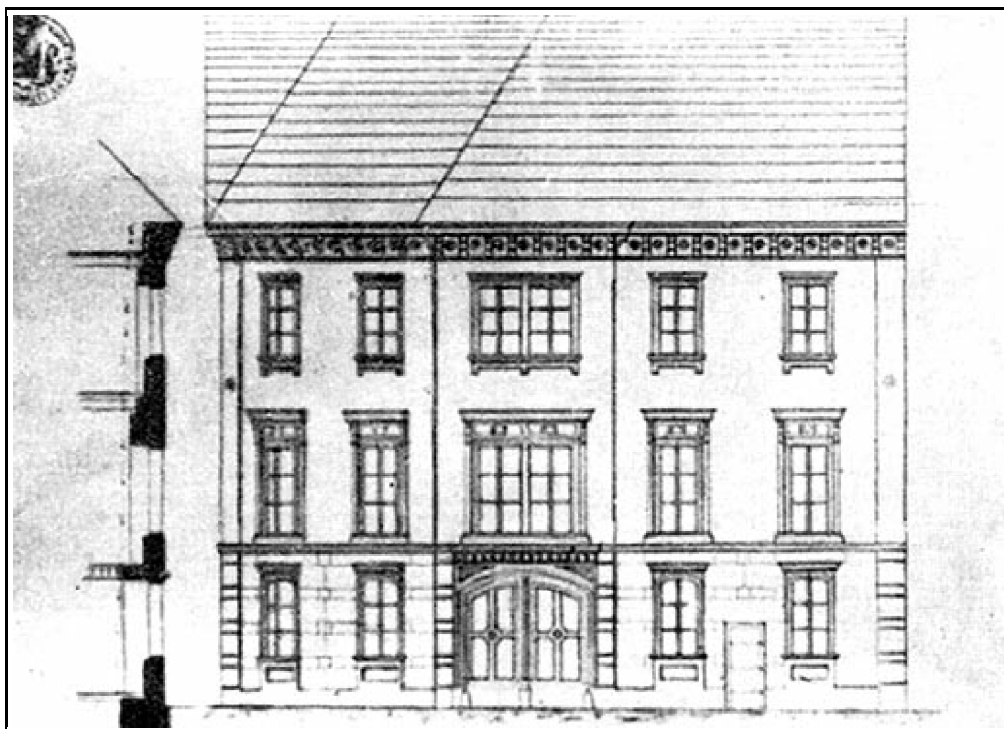
3. Handler József terve a Templom u. 24. sz. ház bővítésére. 1856.
