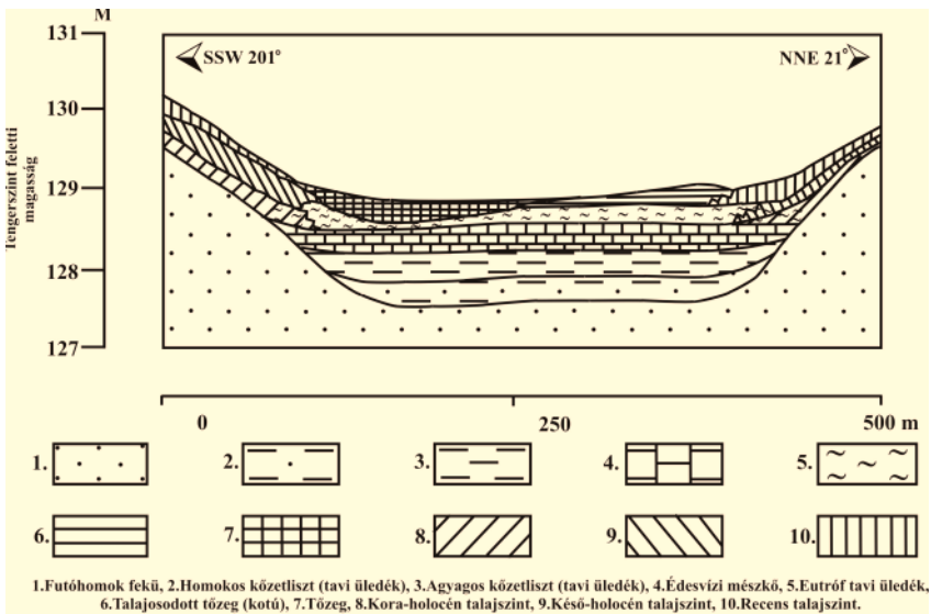
2. ábra A batorligeti láp geológiai keresztsszelvénye (SÜMEGI 1996) Figure 2. The geological cross-section of the Bátorliget-marsh (SÜMEGI 1996)
